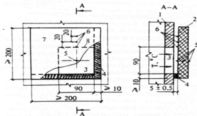
Черт. 1. Схема установки на огневую печь образца вертикальной ограждающей конструкции
