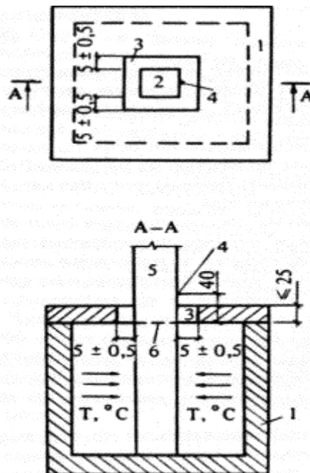
Черт. 3. Схема установки на огневую печь образца вертикальной стержневой конструкции
