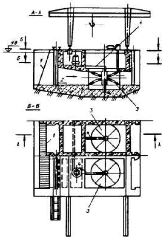
Черт. 9. Конический двухполосный рыбозаградитель с рыбоотводом 1 - сороудерживающая решетка; 2 - камера; 3 - заградитель; 4 - труба рыбоотвода
