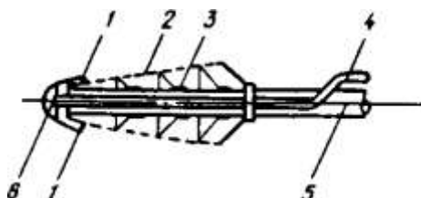
Черт. 7. Сетчатый струереактивный барабан 1 - труба; 2 - промывное устройство; 3 - сетка; 4, 5 - подшипники; 6 - всасывающая линия
