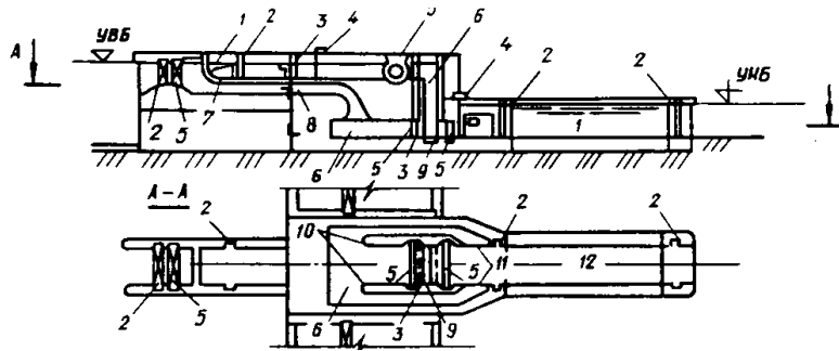
Черт. 5. Рыбоподъемные сооружения. Гидравлический рыбоподъемник 1 - верховой (выходной) лоток; 2 - аварийно-ремонтные заграждения; 3 - сетчатые затворы; 4 - побудительное устройство; 5 - затворы эксплуатационные и блоков питания; 6 - блок питания; 7 - выплывные отверстия; 8 - ихтиологическое устройство; 9 - подъемная площадка; 10 - обходные галереи; 11 - стационарные рыбозащитные решетки; 12 - рыбоаккумулятор
