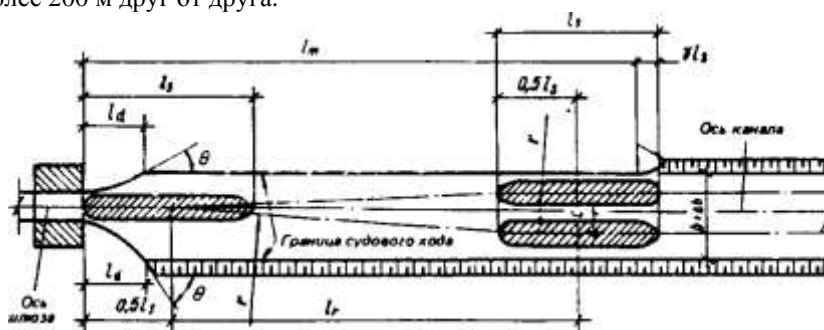
Чертеж. Схема подходного канала к шлюзу для определения длины причальной линии
