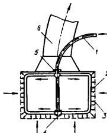
Черт. 7. Сетчатый струереактивный барабан 1 - труба; 2 - промывное устройство; 3 - сетка; 4, 5 - подшипники; 6 - всасывающая линия
