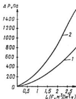
ГРАФИК ДЛЯ ОЦЕНКИ ГЕРМЕТИЧНОСТИ УБЕЖИЩ
