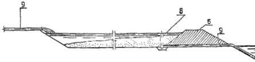
Рис. 4.4. Конструкция береговых отстойников для складирования разработанного земснарядами грунта;
