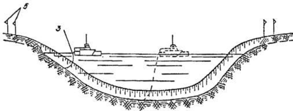
Рис. 9.2. Схема прокладки тягового троса с плавучей площадки:
