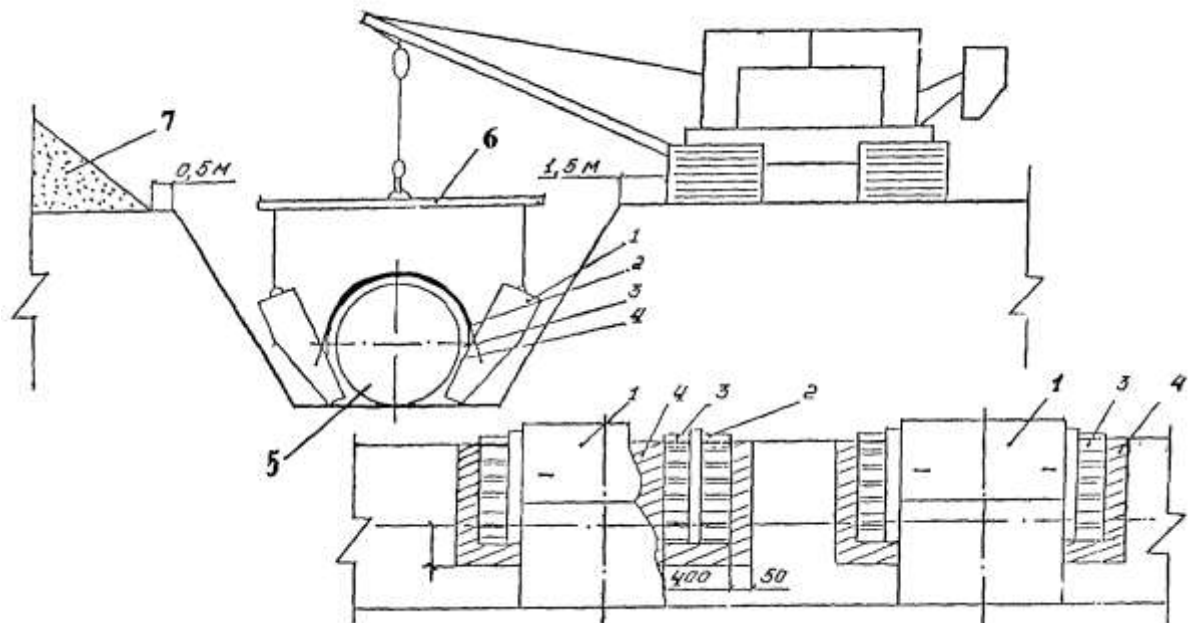
Рис 7.1. Схема балластировки трубопровода утяжелителями УБО:
