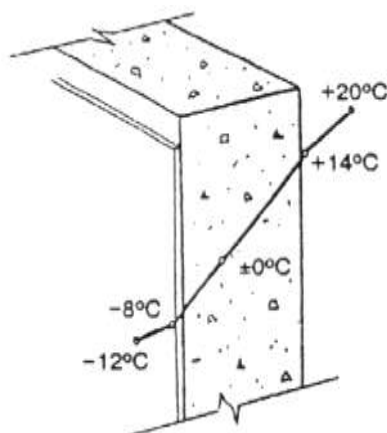
б) Наружная стена с теплоизоляцией толщиной 75 мм
