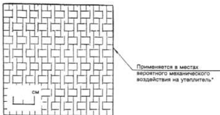
Рисунок А3 — Обычная арматурная сетка из стекловолокна
