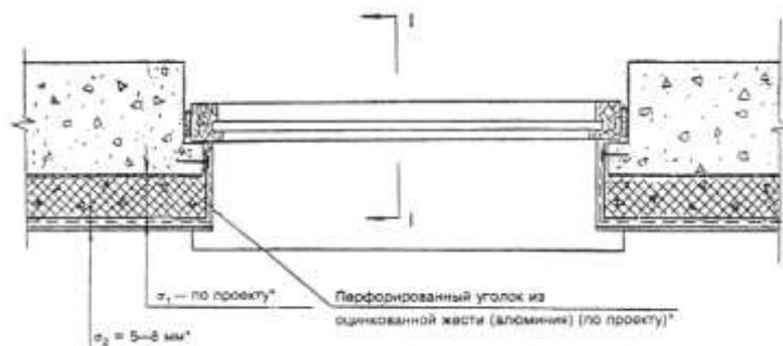
Рисунок А13 — Фрагмент примыкания наружной теплоизоляции здания к карнизной плите
