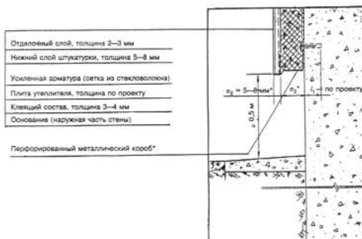
Рисунок А8 — Фрагмент наружной теплоизоляции здания с тонкой штукатуркой по утеплителю
