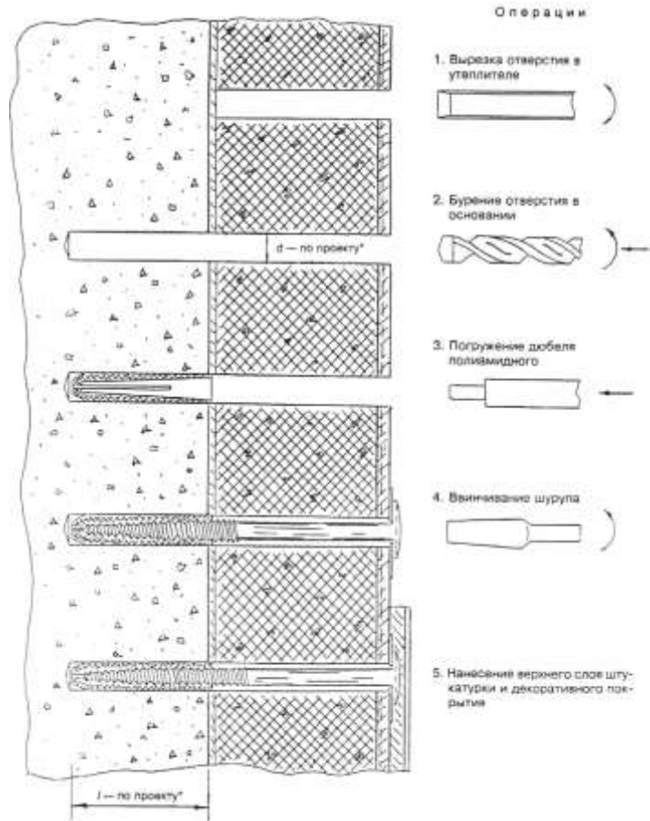
Рисунок А6 — Крепление плиты утеплителя с помощью дюбеля полиамидного и шурупа
