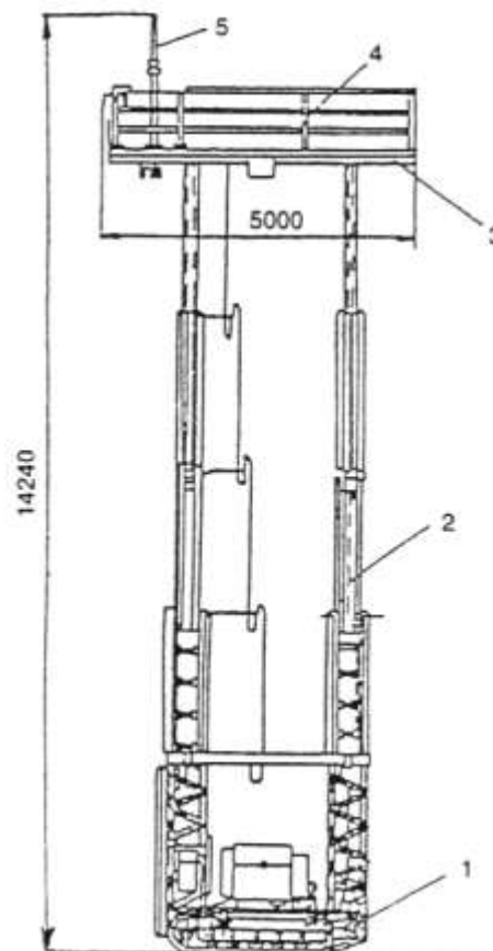
Подмости ПВС-12
