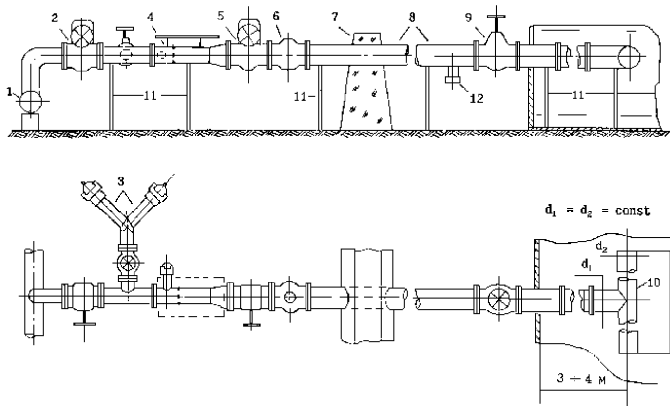
Рис. 1. Принципиальная схема стационарной системы подслоного тушения пожаров горючих жидкостей в резервуарах (ССПТ) 1 - сухотруб ССПТ; 2, 5 - электрозадвижки; 3 - разветвление для подключения передвижной пожарной техники; 4 - высоконапорный генератор пены со смесителем-дозатором и защитным кожухом; 6 - обратный клапан; 7 - обвалование; 8 - пенопровод; 9-задвижка; 10 - пенослив; 11 - опоры; 12 - сливной патрубков.
