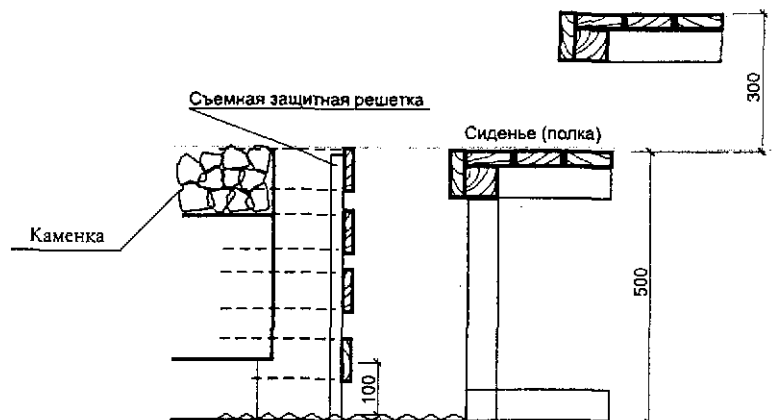
Рис. 6.2 Варианты решений и оборудование саун
