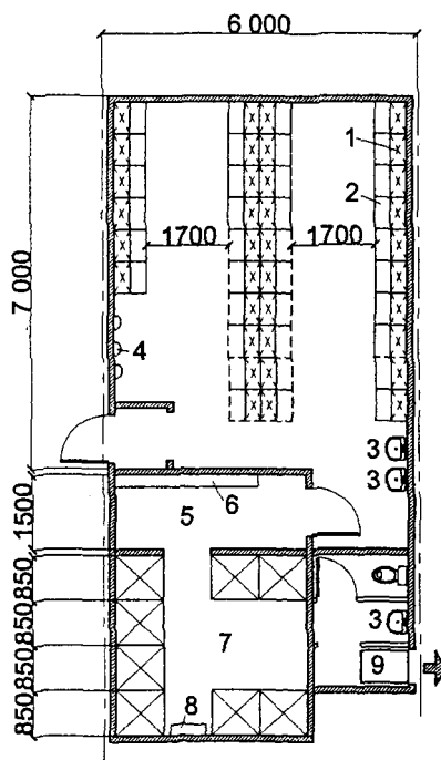
1 - двухъярусные закрытые шкафы; 2 - скамьи для переодевания; 3 - умывальник; 4 - сушилка для волос; 5 - преддушевая; 6 - вешалка для полотенец; 7 - душевая; 8 - стеллаж для мыла; 9 - ножной проходной душ
