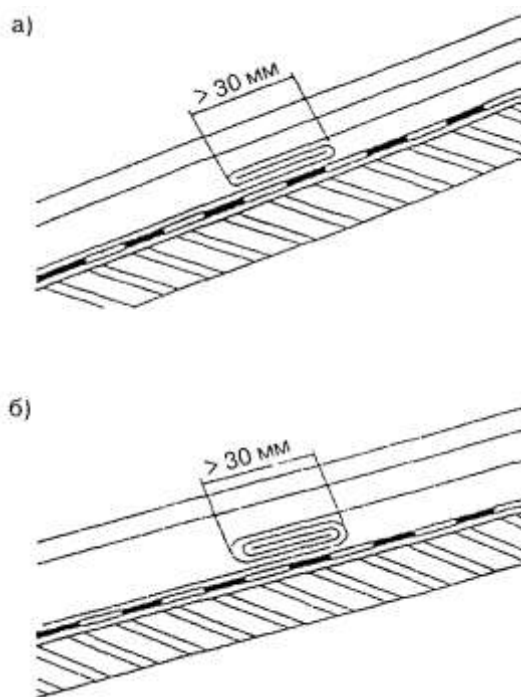
а — одинарный; б — двойной
