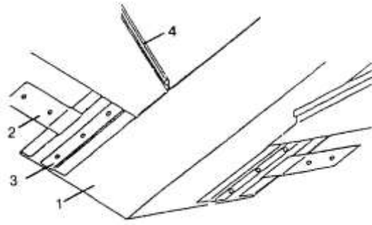
1 — картина разжелобка; 2 — медный кляммер; 3 — фасонный дополнительный медный кляммер; 4 — двойной стоячий фальц с квадратными кромками
