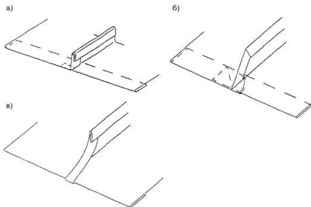
Рисунок 14 — Формы стоячего фальца у карниза
