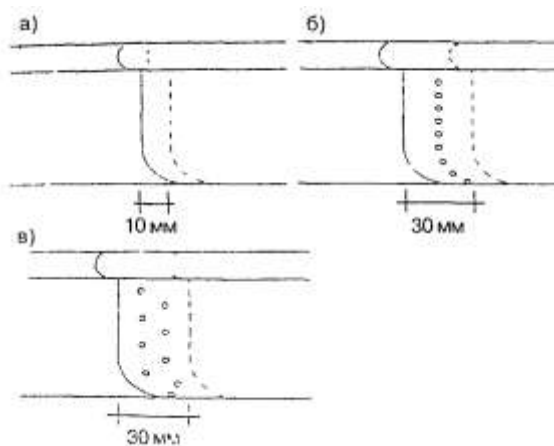
а — мягкая пайка или твердая сварка; б — мягкая сварка с одним рядом заклепок; в — мягкая сварка с заклепками, расположенными в шахматном порядке
