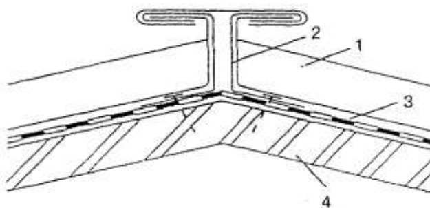
Рисунок 18 — Конек без вентиляционных зазоров
