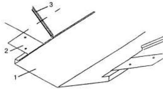
1 — картина разжелобка; 2 — медный кляммер; 3 — двойной стоячий фальц с квадратными кромками
