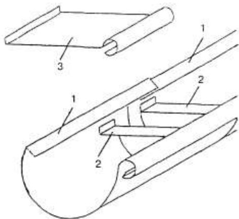
1 — полукруглый желоб; 2 — ограничитель; 3 — медная покрывающая полоса
