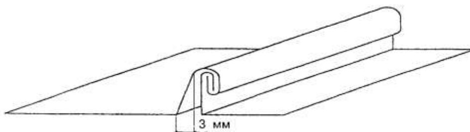
Рисунок 4 — Двойной фальц с компенсационным стыком
