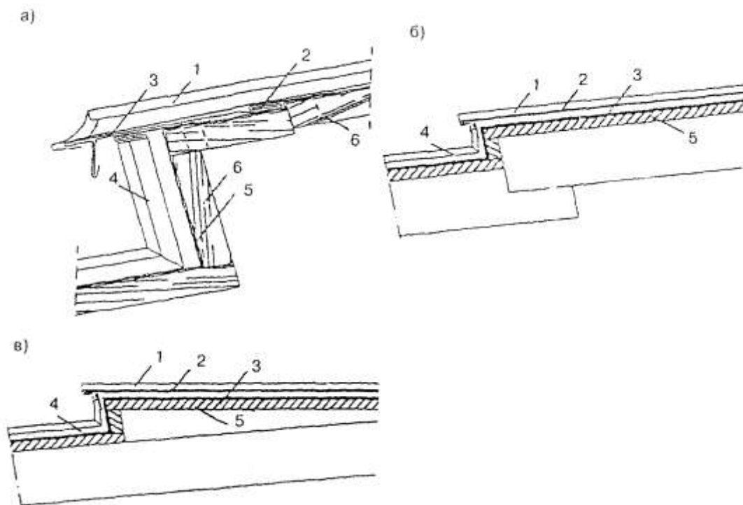
а: 1 — стоячий фальц со скошенными кромками; 2 — лежащий фальц со сплошным кляммером; 3 — карнизный свес; 4 — фальцевая медная кровля; 5 — подстилающий слой; 6 — основание под кровлю; б, в: 1 — стоячий фальц с квадратными кромками; 2 — карнизный свес; 3 — подстилающий слой; 4 — фальцевая медная кровля; 5 — основание под кровлю
