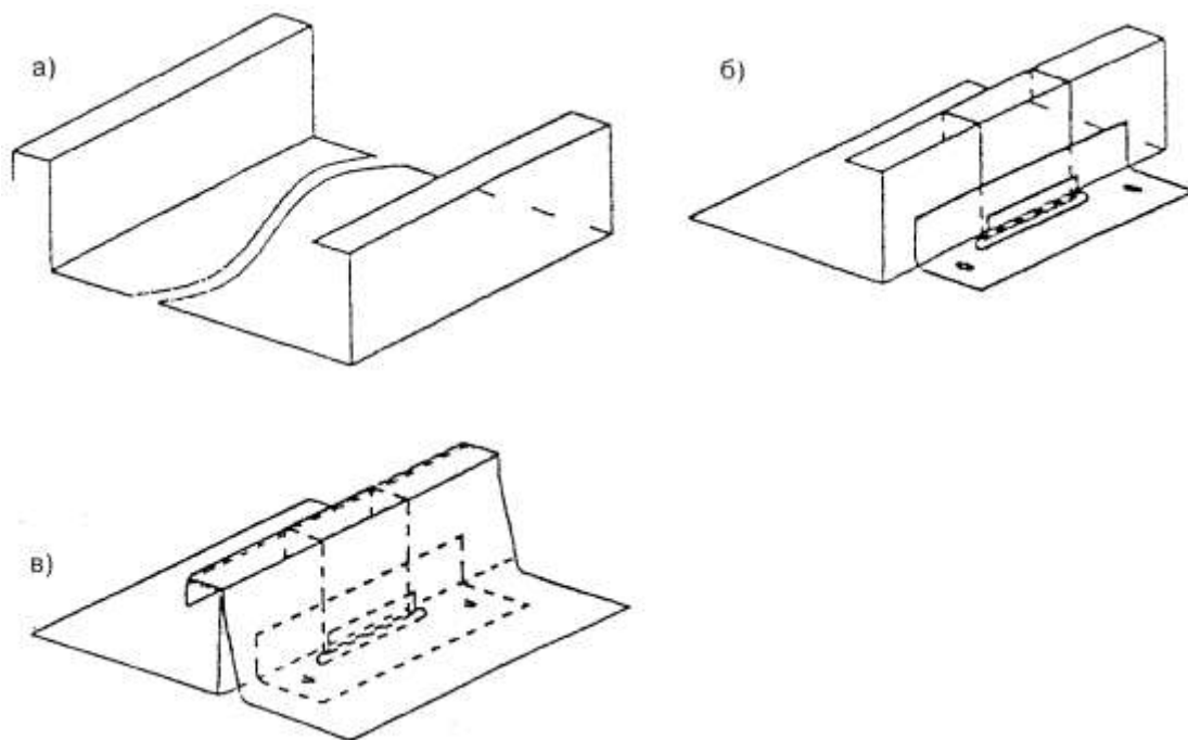
а — устройство кромок на листе; б — установка кляммера (скользящего кляммера) на основание и кромку листа; в — установка второго листа с отогнутой кромкой
