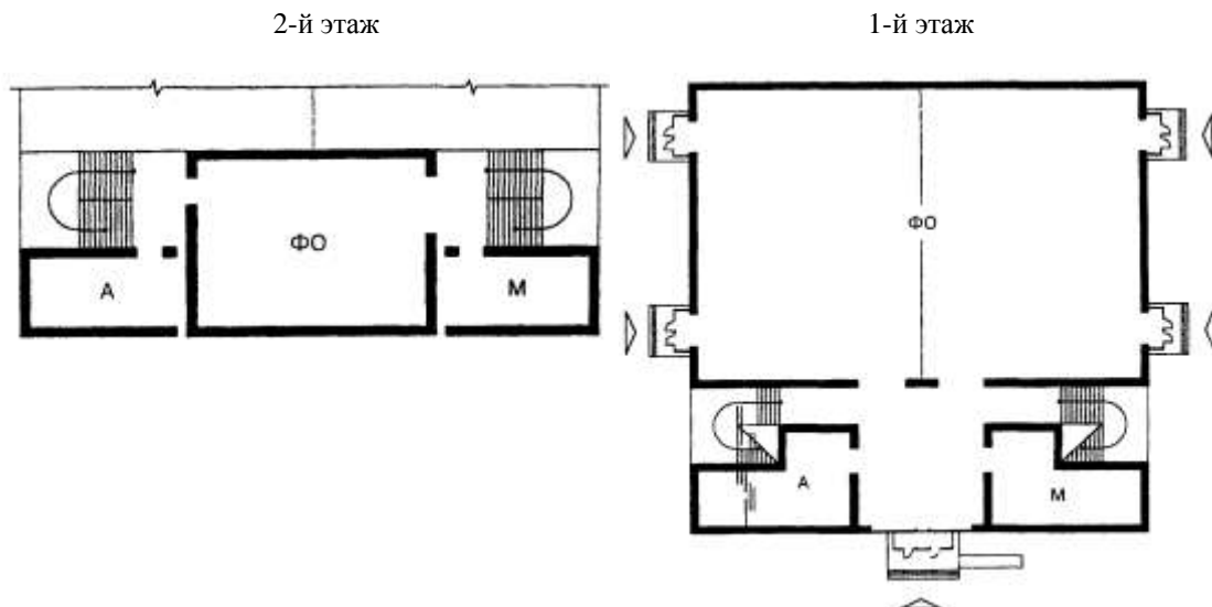
Рисунок Б.2 - Проектное решение досугово-оздоровительного центра
