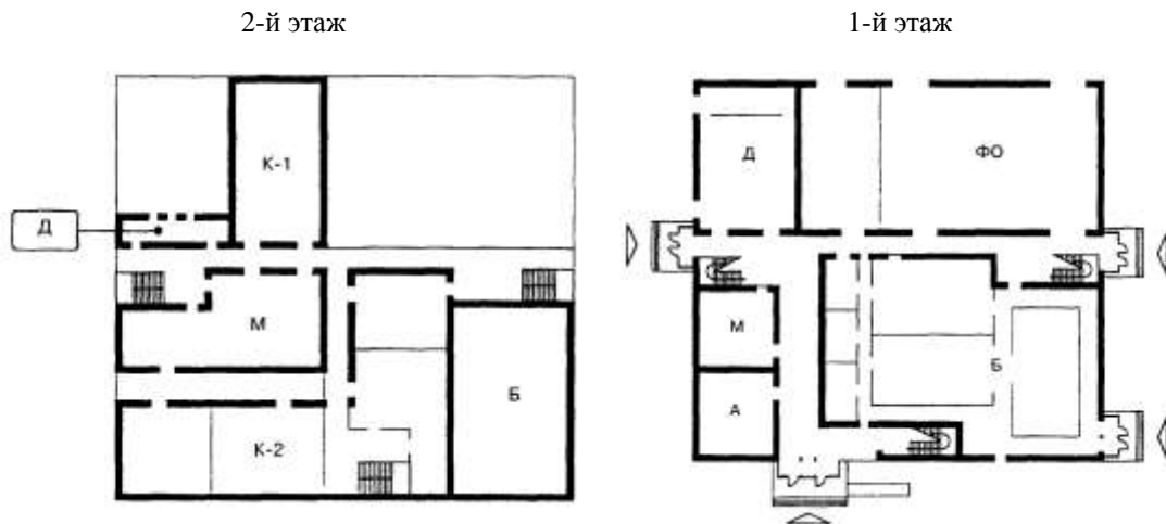
Рисунок Б.1 - Приспособление здания школы под досугово-оздоровительный центр (типовой проект 224-01-686.90)
