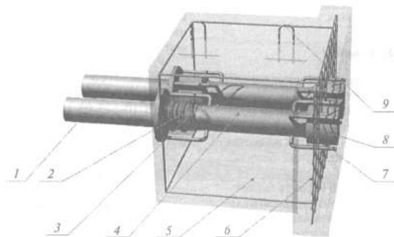
Рисунок 1 — Узел ответвления стального трубопровода D_v = 150 мм налево от асбестоцементного D_v = 200 мм
