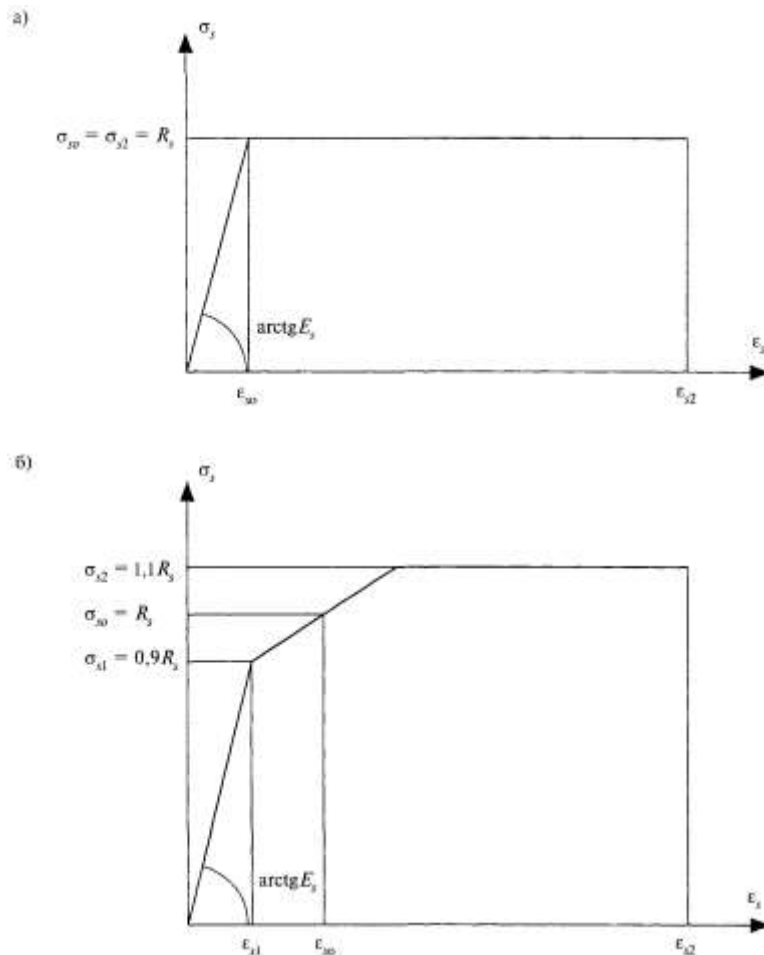
a - двухлинейная; б – трехлинейная Рисунок 2 - Диаграммы состояния растянутой арматуры
