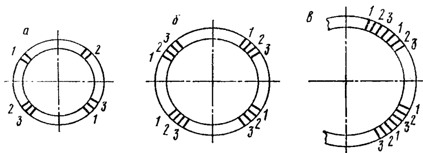
Рис.3 - Схема вырезки образцов для механических испытаний
