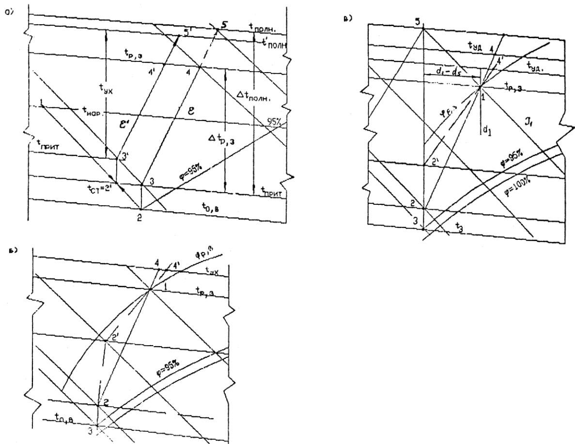
Рис. 1. Схемы процессов приготовления приточного воздуха, построение на J - d диаграмме:
