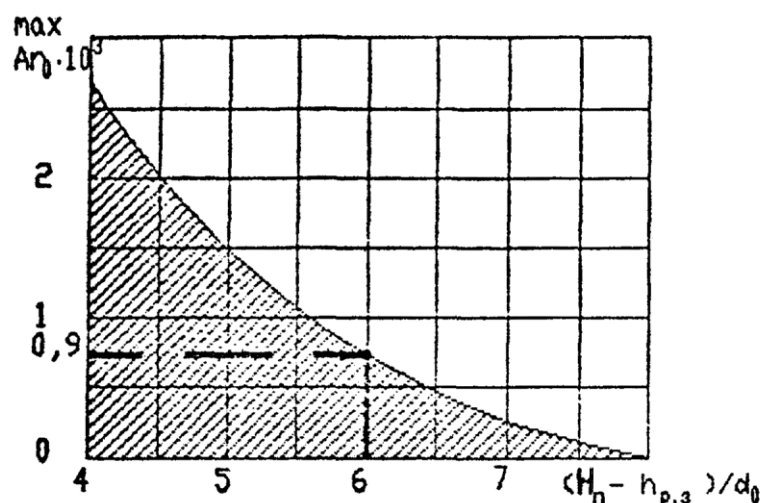
Рис. 4. Предельное значение критерия Архимеда Ar_0 , при котором сохраняется расчетная схема развития струи.
