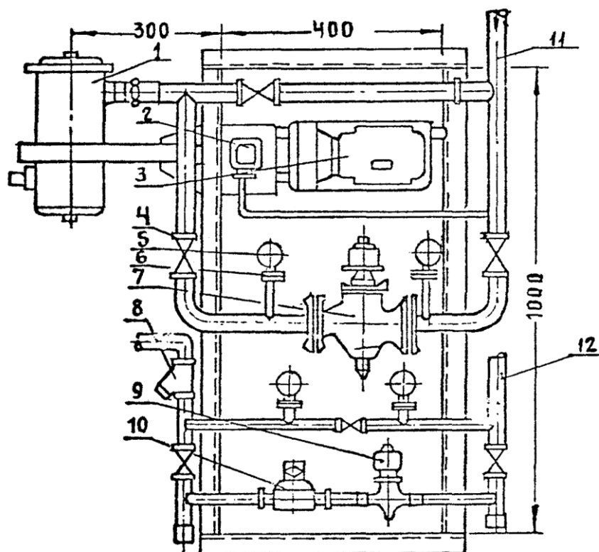
Рис. 5. Пример компоновки щита управления установки «Туман»:
