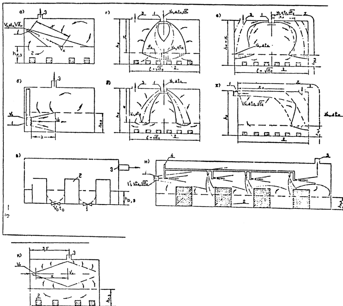
Рисунок 2. Способы подачи воздуха в производственные помещения:
