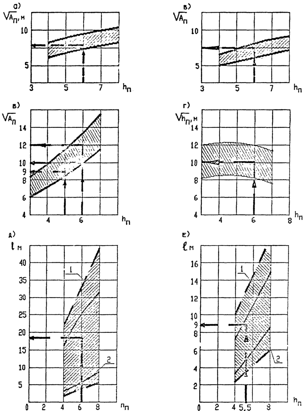
Рис. 3. Максимальный размер помещения или его зоны l = \sqrt{A_n} , м;
