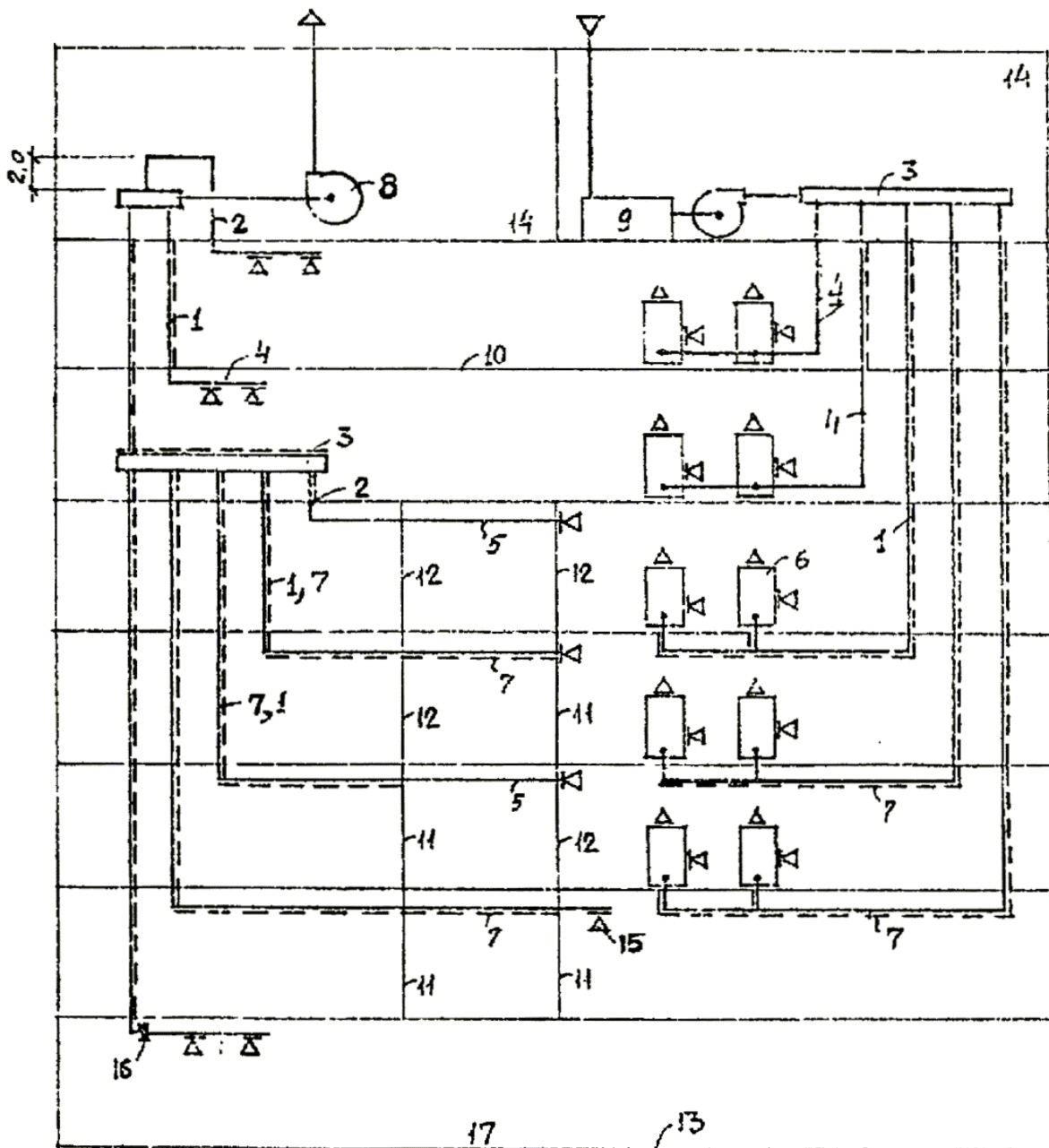
Рис. 2. Схемы воздухопроводов с горизонтальными коллекторами.
