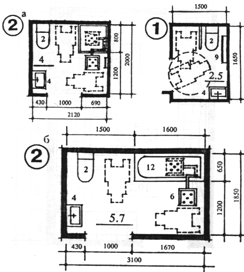
Рис. 6. Планировочные схемы санитарных узлов. Вариант 1 — уборная с умывальником. Вариант 2 — санитарный узел при спальном комнате. (а — вариант с душем, б — вариант с ванной). Экспликация оборудования: 1 — унитаз детский 30х50, 2 — унитаз для взрослых 40х60, 3 — умывальник детский 50х30, 4 — умывальник для взрослых 60х40, 5 — душевой поддон 80х80, 6 — поворотное кресло, 7 — ногомойка 40х60, 8 — банкетка 40х40, 9 — вешалка для полотенец, 10 — поручни-держатели, 11 — шкаф хозяйственный
