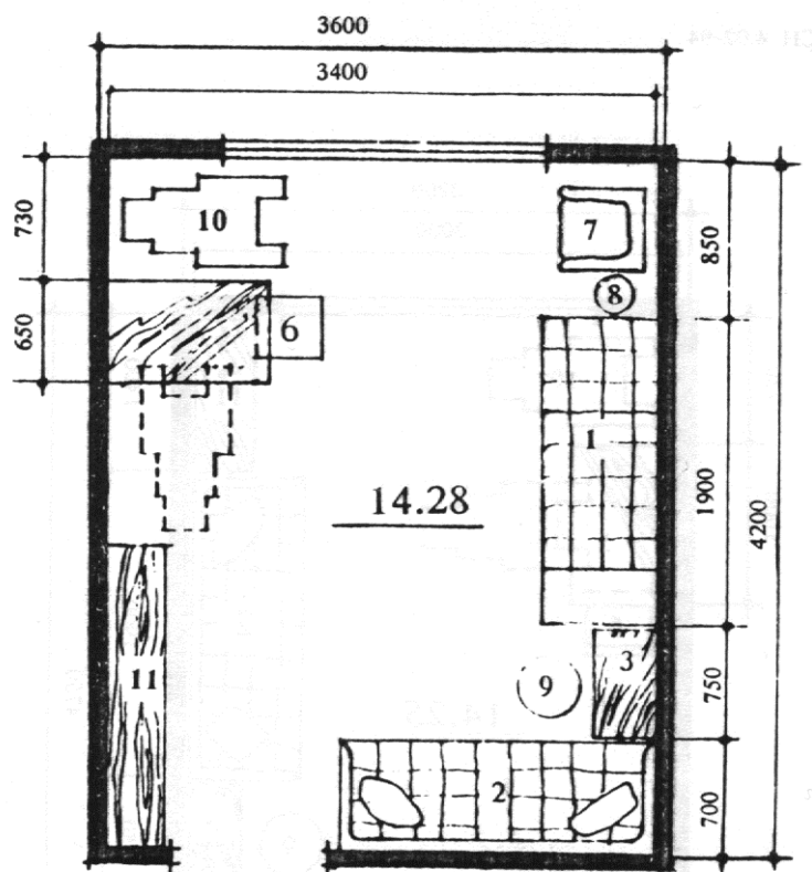
Рис. 1. Планировочная схема спальни на 2 места. (Вариант при шаге 3,6 м). Экспликация оборудования: 1 — кровать 190х70, 2 — диван 200х75, 3 — тумбочка 40х80, 4 — тумбочка 40х40, 5 — стол 60х100, 6 — стул 40х40, 7 — кресло 50х50, 8 — торшер, 9 — банкетка, 10 — инвалидная коляска, 11 — комбинированный шкаф
