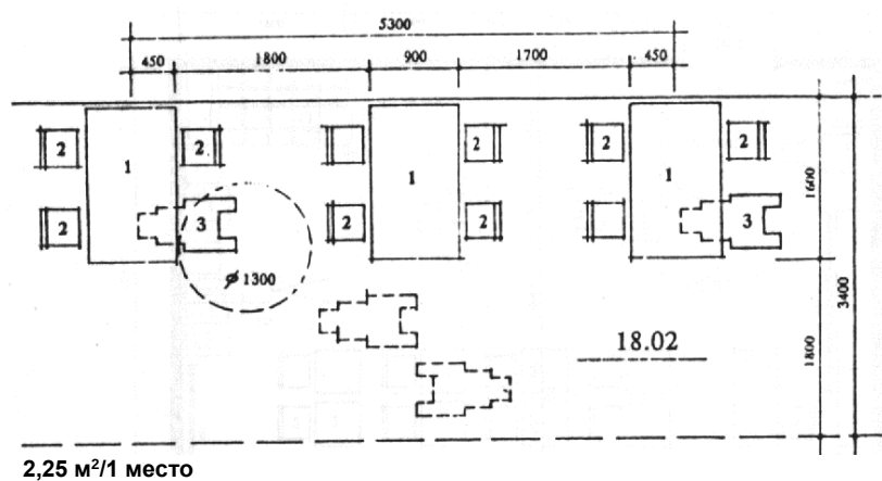
Рис. 10. Габаритная схема организации обеденного места в общей комнате при семейном проживании: вариант 1 — на 8 чел. Экспликация оборудования: 1 — стол, 2 — стул, 3 — инвалидная коляска
