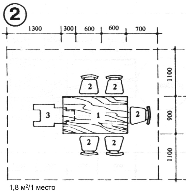
Рис. 12. Схема организации обеденного места в общей комнате при семейном проживании. Вариант 2 на 6 чел. Экспликацию оборудования см. рис. 10
