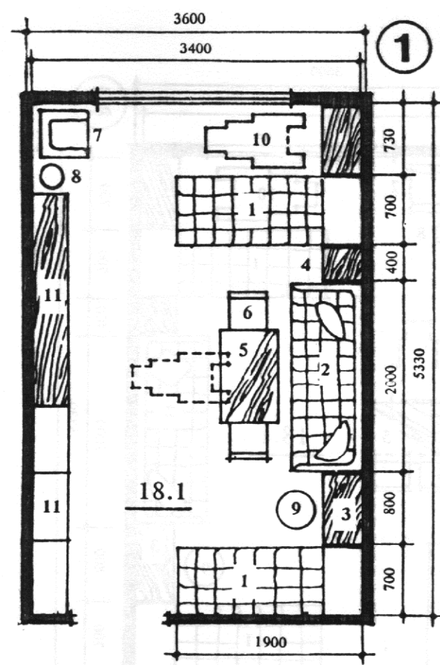
Рис. 3. Планировочная схема спальни на 3 места (вариант 1). Экспликацию оборудования см. рис. 1
