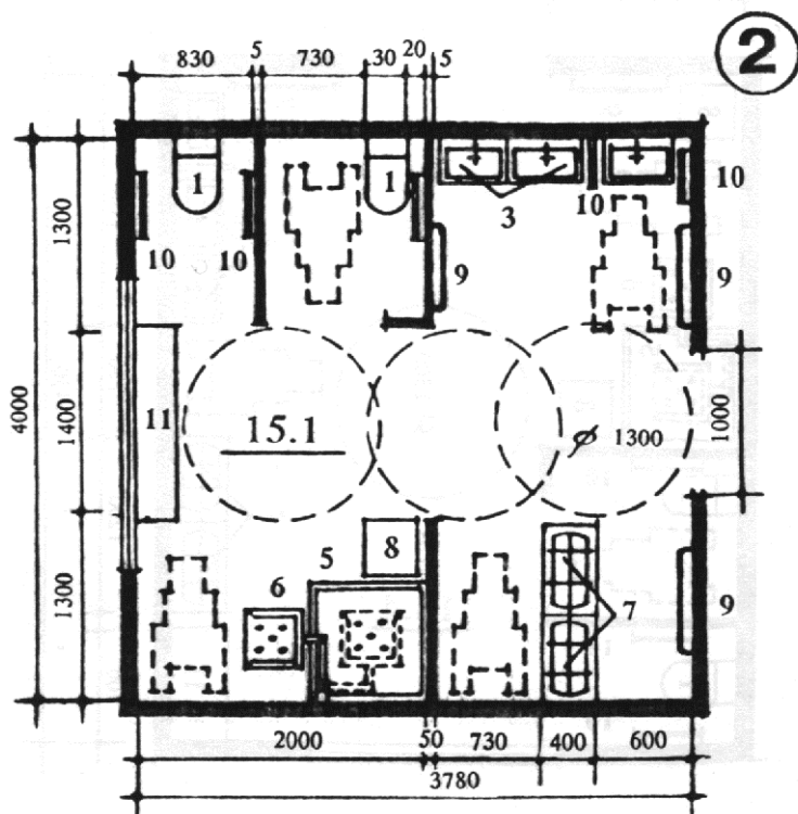
Рис. 8. Планировочная схема санитарного узла для дошкольных групп (вариант 2). Экспликацию оборудования см. рис. 7
