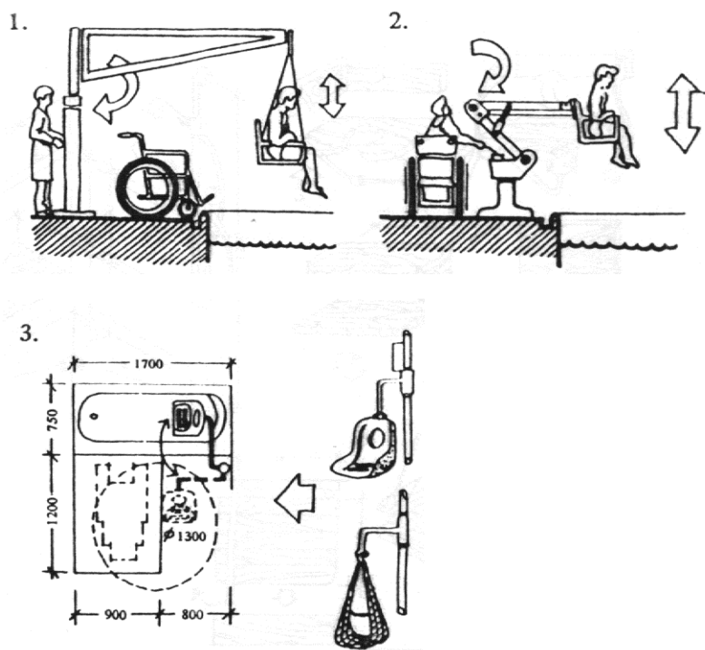
Рис. 13. Примеры оборудования санитарно-гигиенических помещений. Зарубежный опыт (Х. Ю. Калмет)
