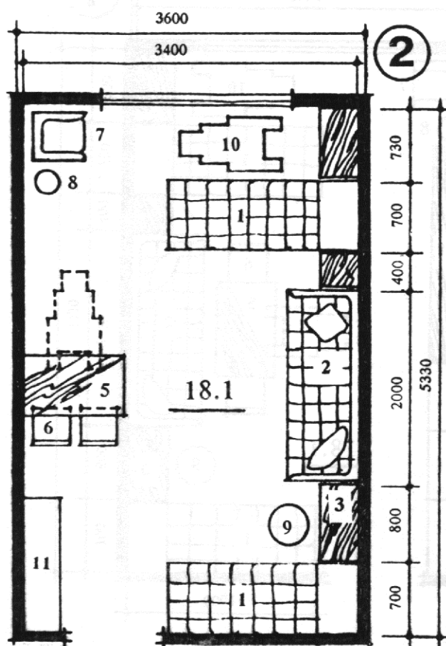
Рис. 4. Планировочная схема спальни на 3 места (вариант 2). Экспликацию оборудования см. рис. 1
