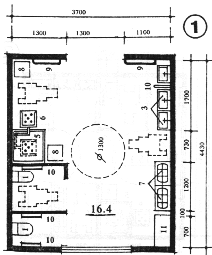
Рис. 7. Планировочная схема санитарного узла для дошкольных групп (Вариант 1). Экспликация оборудования: 1 — унитаз детский 30х50, 2 — унитаз для взрослых 40х60, 3 — умывальник детский 50х30, 4 — умывальник для взрослых 60х40, 5 — душевой поддон 80х80, 6 — поворотное кресло, 7 — ногомойка 40х60, 8 — банкетка 40х40, 9 — вешалка для полотенец, 10 — поручни-держатели, 11 — шкаф хозяйственный
