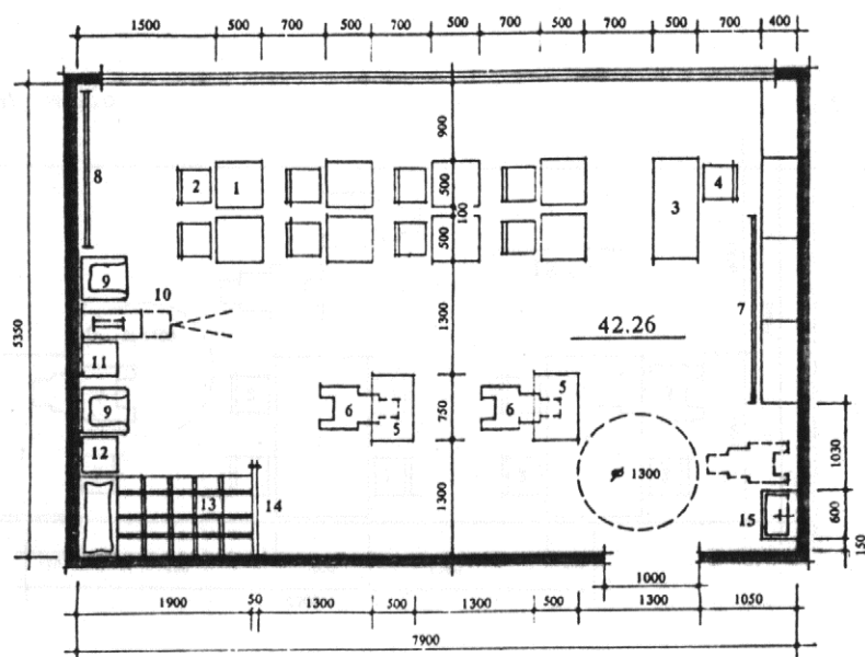
Рис. 9. Планировочные схемы класса на 10 чел. с зоной психологической разгрузки. Экспликация оборудования: 1 — стол ученический, 2 — стул ученический, 3 — стол учителя, 4 — стул учителя, 5 — стол ученический для инвалида-колясочника, 6 — инвалидная коляска, 7 — доска, 8 — шведская стенка, 9 — кресло, 10 — кинопроекторный аппарат, 11 — табурет, 12 — тумбочка, 13 — кушетка, 14 — экран, 15 — умывальник
