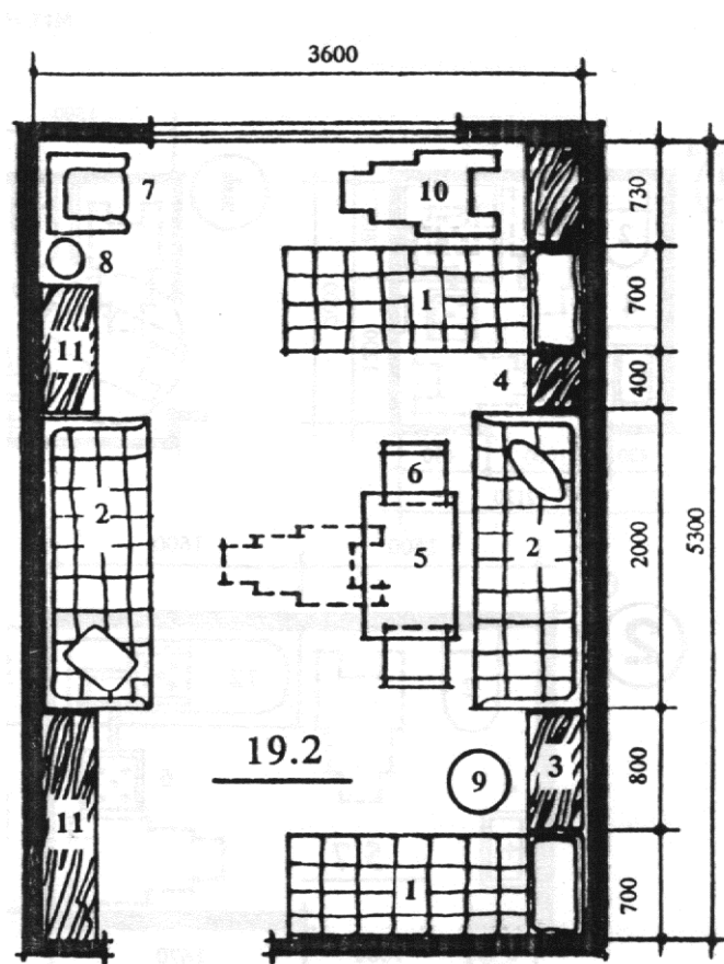
Рис. 5. Планировочная схема спальни на 4 места. Эспликацию оборудования см. рис. 1
