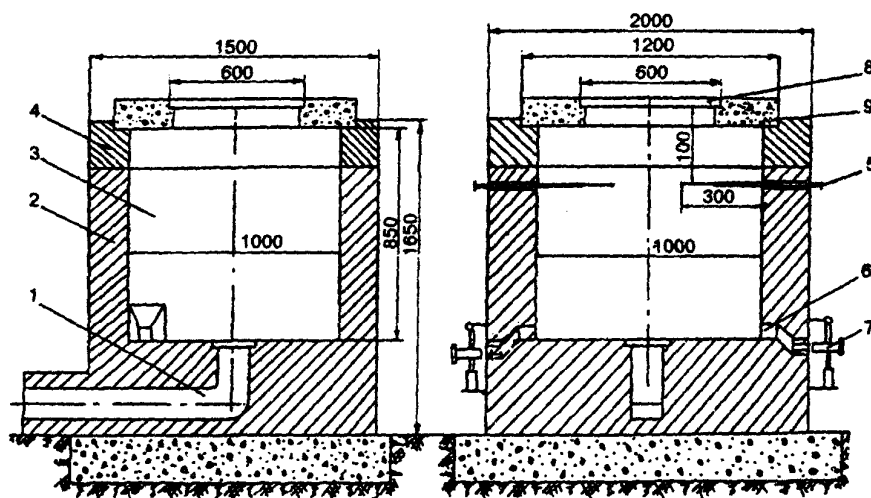
Рисунок 3 - Установка для теплофизических исследований и испытаний малогабаритных фрагментов плоских конструкций и отдельных узлов их стыковых сопряжений и креплений.
