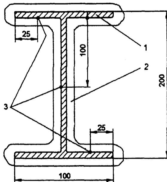
Рисунок 2 - Схема расстановки термоэлектрических преобразователей в среднем сечении на поверхности испытанного образца
