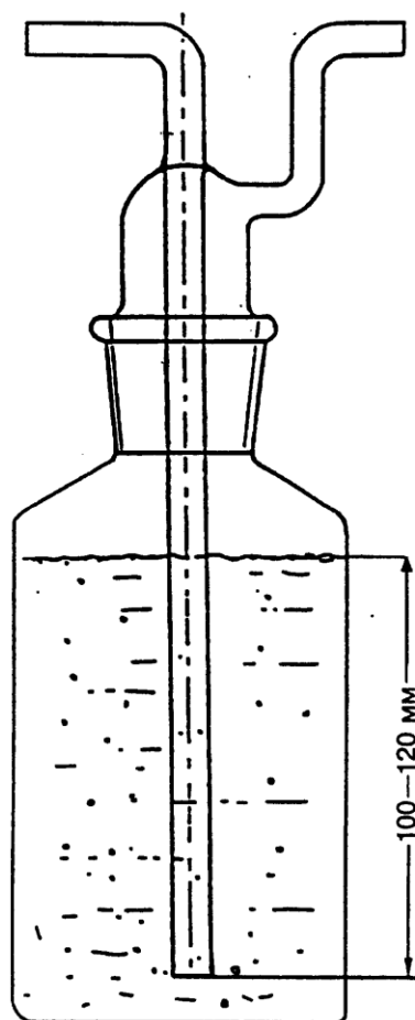
Рисунок 2 - Сосуд-смеситель
