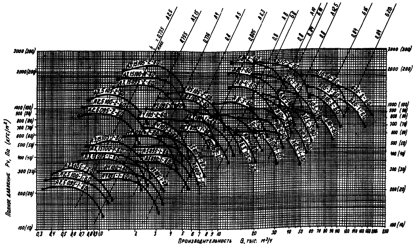
Рис. I. Сводный график для подбора вентиляторов при работе с частотой тока 60 Гц
