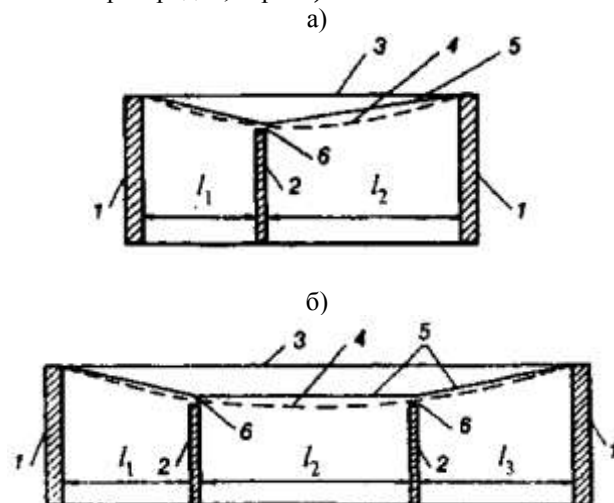
Черт. 4. Схемы для определения значений l ( l_1, l_2, l_3 ) при наличии между стенами капитальных перегородок
