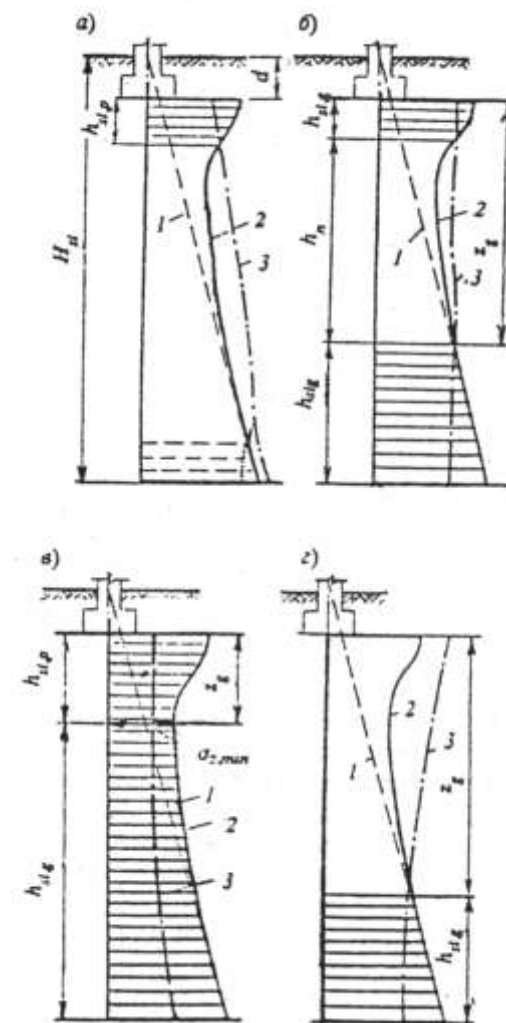
Рис. 4. Схемы к расчету просадок основания
