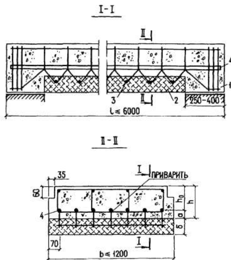
Черт. 10. Конструкция нагибаемого железобетонного элемента, нагреваемого до температуры более 400 °С со стороны растянутой зоны 1 - тяжелый жаростойкий бетон; 2 - теплоизоляционный слой из легкого жаростойкого бетона; 3 - сетка из жаростойкой стали диаметром 4 мм; 4 - продольная рабочая арматура
