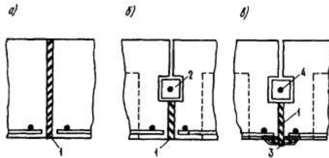
Черт. 8. Температурные швы в конструкциях из жаростойкого бетона а - шов, заполненный шнуровым асбестом; б - то же, с бетонным брусом; в - то же, с металлическим компенсатором;
