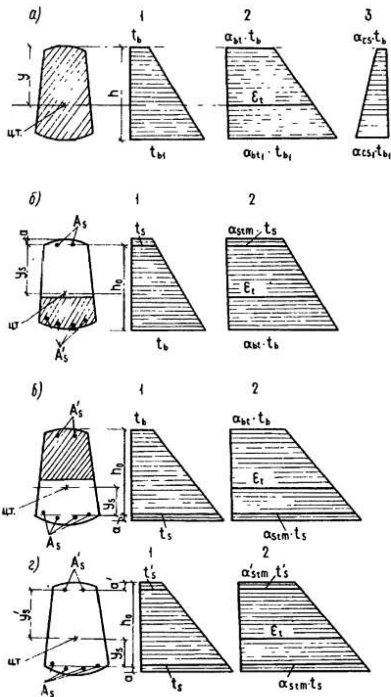
Черт. 3. Схемы распределения температур (1) и деформаций от неравномерного нагрева (2) и остывания (3) при прямолинейном изменении температур по высоте сечения элемента а - бетонного и железобетонного без трещин; б - железобетонного с трещинами в растянутой зоне, расположенной у менее нагретой грани; в - то же, у более нагретой грани; з - железобетонного с трещинами по всей высоте сечения
