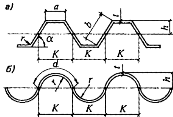
Черт. 13. Геометрические параметры для гофра
