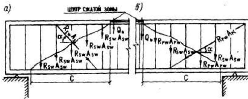
Черт. 7. Схема усилий в сечении, наклонном к продольной оси железобетонного элемента, при расчете его по прочности на действие поперечной силы а — с ненапрягаемой арматурой; б — с напрягаемой арматурой
