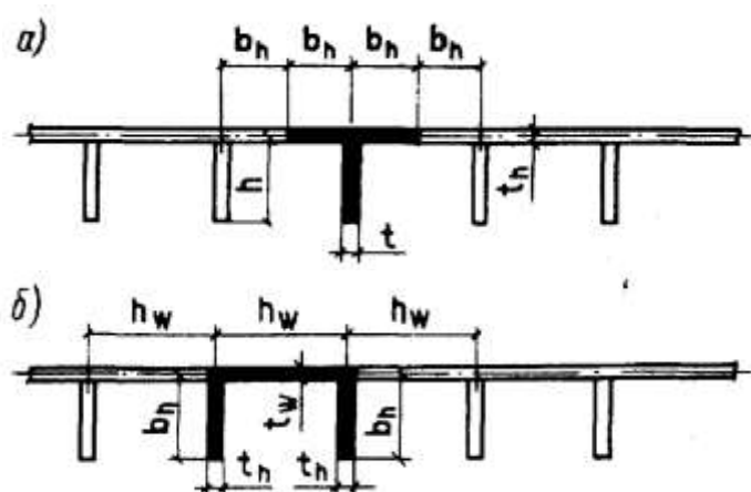
Черт. 12. Схемы расчетных сечений пластинок ортотропных плит
