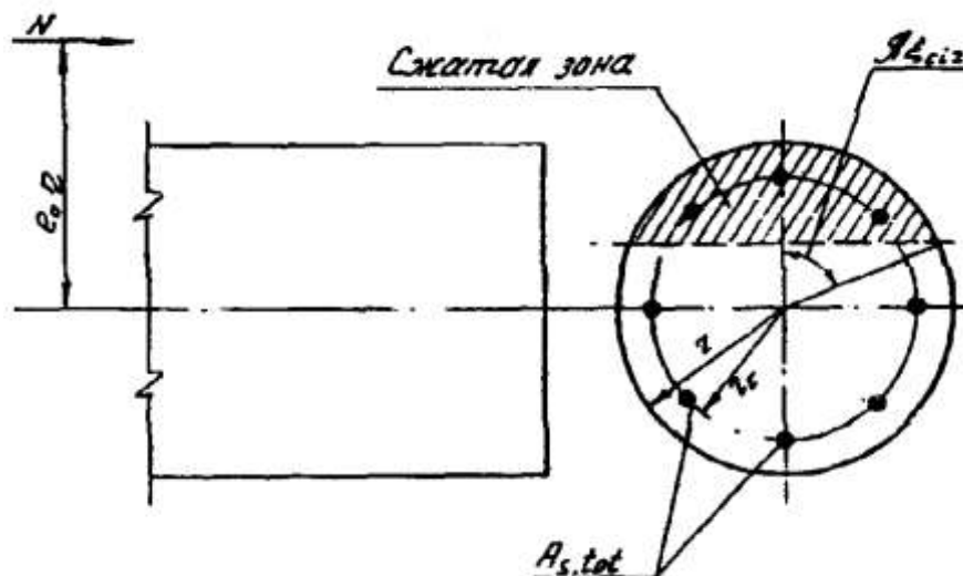
Чертеж. Схема, принимаемая при расчете круглого сечения внецентренно сжатого элемента
