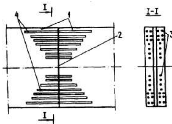
Черт. 18. Клеештыревой стык 1 — стыкуемые блоки; 2 — стык блоков; 3 — отверстия для штырей; 4 — вклеенные в отверстия штыри
