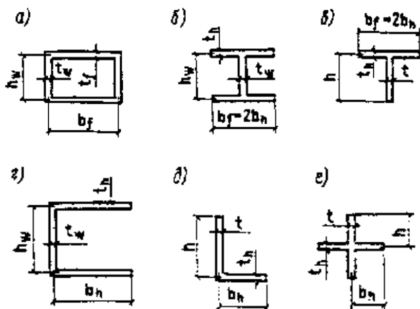
Черт. 11. Схемы расчетных сечений элементов, не подкрепленных ребрами жесткости
