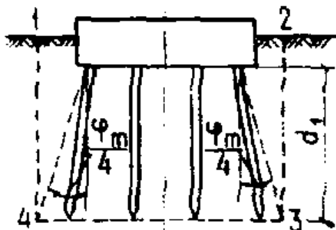
Черт. 1. Условный свайный фундамент с ростверком, заглубленным в грунт при угле наклона свай менее \varphi_m/4
