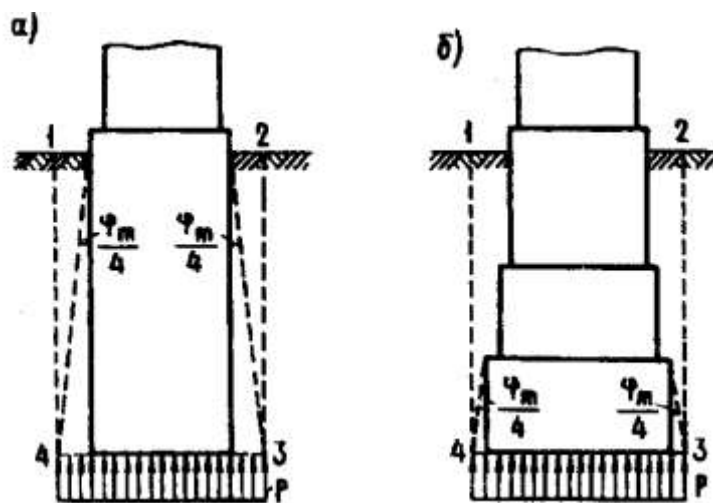
Черт. 5. Условный фундамент из опускающего колодца а — без уступов; б — с уступами
