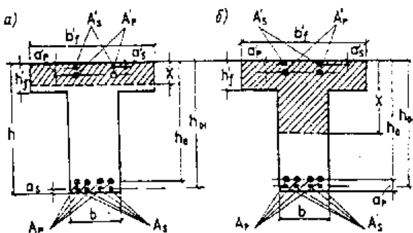
Черт. 3. Форма сжатой зоны в сечениях железобетонных элементов с плитой в сжатой зоне а — при расположении границы сжатой зоны в плите; б — то же, в ребре
