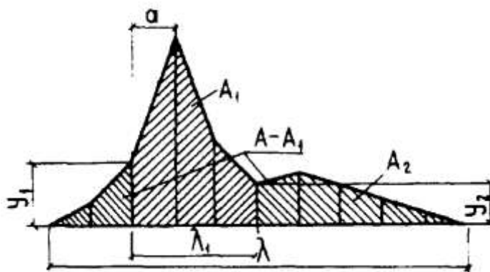
Черт. 2. Часть линии влияния длиной \lambda , включая ее вершину
