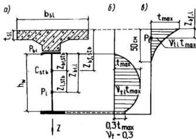
Черт. 14. Поперечное сечение сталежелезобетонной конструкции и расчетные эпюры разности температур а — схема поперечного сечения; б — криволинейная эпюра разности температур по высоте стальной части сечения; в — криволинейная эпюра разности температур для верхней части сечения балки
