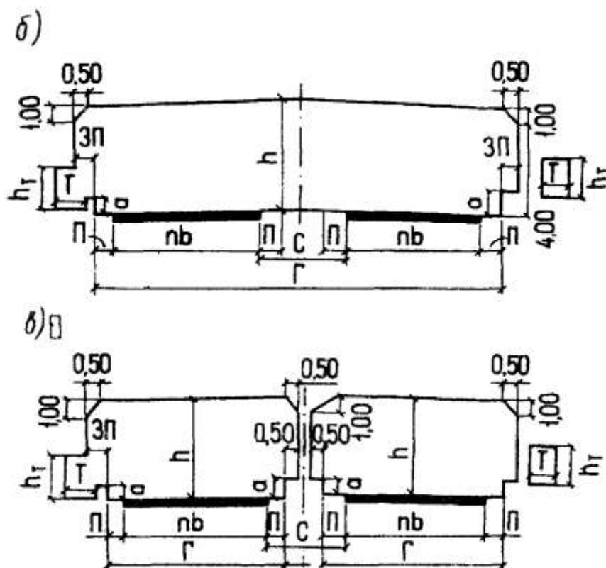
Черт. 1. Схемы габаритов приближения конструкций на автодорожных и городских мостах
