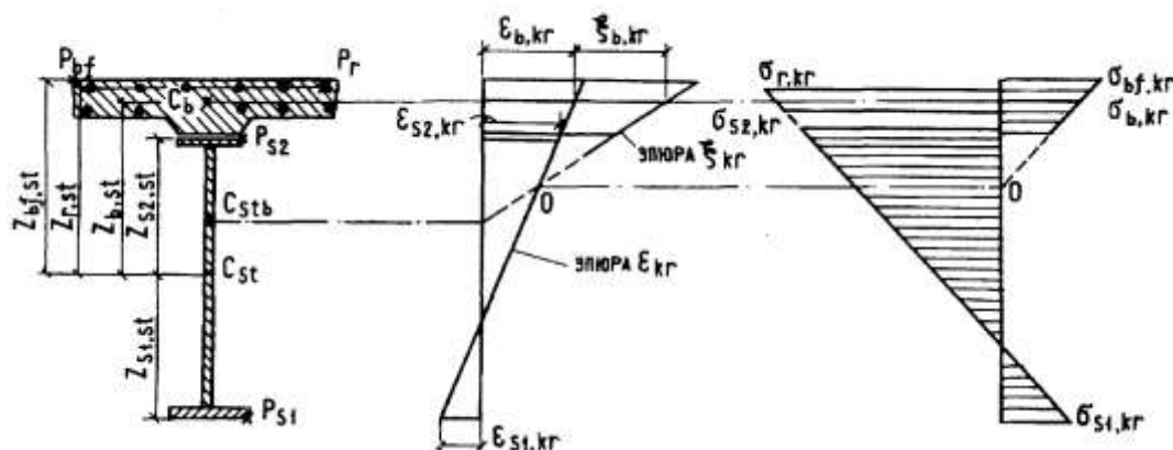
Эпюры относительных деформаций и внутренних напряжений от ползучести бетона
