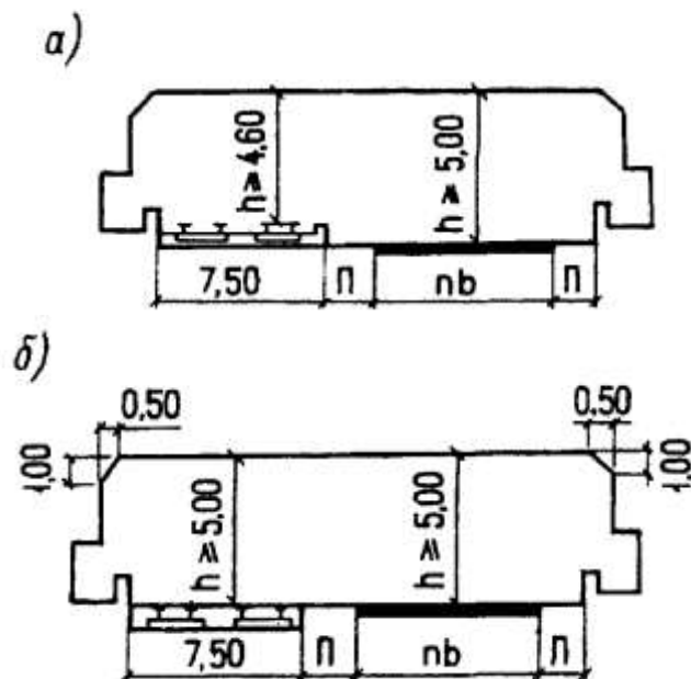
Черт. 2. Схемы габаритов приближения конструкций на городских мостах с трамвайным движением
