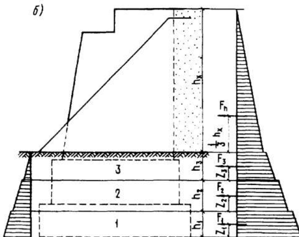
Схема эпюр давления грунта на опоры моста для определения равнодействующей нормативного горизонтального (бокового) давления на опоры
