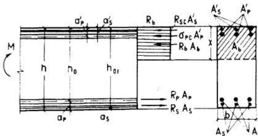
Черт. 2. Схема усилий и эпюра напряжений в сечении, нормальном к продольной оси изгибаемого железобетонного элемента, при расчете его по прочности
