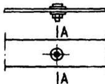
Черт. 1. Расположение проверяемого на выносливость расчетного сечения А—А по основному металлу в сечениях нетто по соединительным болтам составных элементов, а также у свободного отверстия
