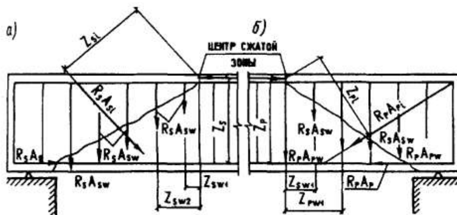
Черт. 8. Схема усилий в сечении, наклонном к продольной оси железобетонного элемента, при расчете его по прочности на действие изгибающего момента а — с ненапрягаемой арматурой; б — с напрягаемой арматурой
