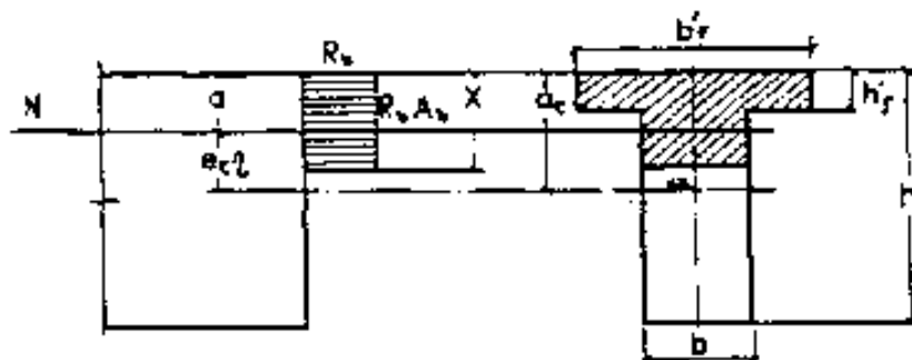
Черт. 4. Схема усилий и эпюра напряжений в сечении, нормальном к продольной оси внецентренно сжатого бетонного элемента
