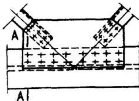
Черт. 3. Расположение проверяемого на выносливость расчетного сечения А—А по основному металлу в сечении брутто по первому ряду высокопрочных болтов в прикреплении фанонки к нестыкуемым в данном узле поясам сплошных балок и элементам решетчатых форм
