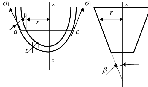
Рис. 17. Схема оболочки вращения Рис. 18. Схема конической оболочки вращения
