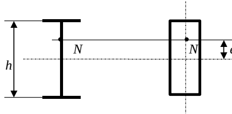
Рис. 16*. Схема внецентренно-сжатых элементов двутаврового и коробчатого сечений
