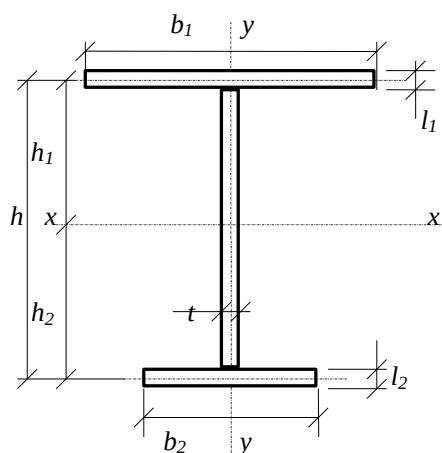
Рис. 28. Схема двутаврового сечения с одной осью симметрии при изгибе
