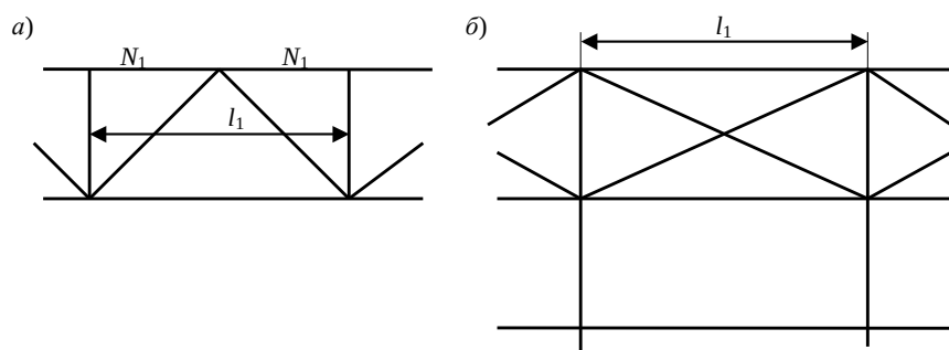
Рис. 8. Схемы для определения расчетной длины пояса фермы из плоскости а – схема фермы; б – схема связей между фермами (вид сверху)
