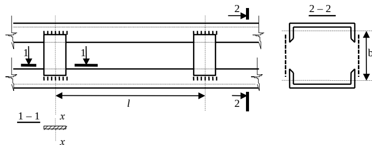
Рис. 3. Составной стержень на планках
