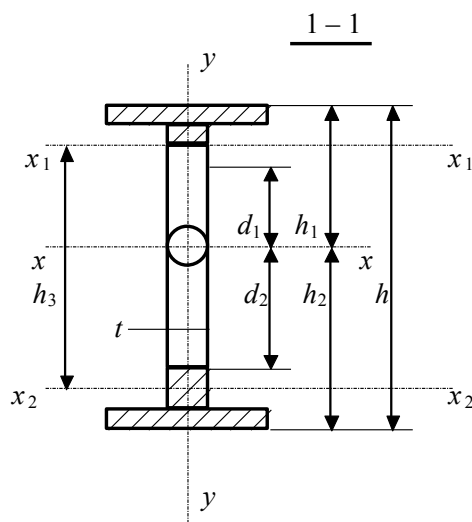
Рис. 23. Схема участка балки с перфорированной стенкой
