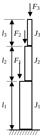
Рис. 25. Схема двухступенчатой колонны
