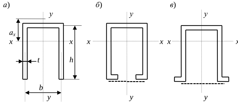
Рис. 1. П-образные сечения элементов а – открытое; б, в – укрепленные планками или решеткой
