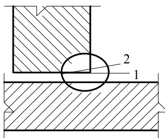
Рис. 20. Схема расчетных сечений сварного соединения с угловым швом 1 – сечение по металлу шва; 2 – сечение по металлу границы сплавления
