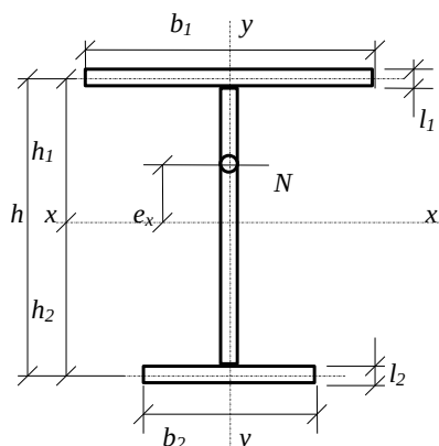
Рис. 27. Схема двутаврового сечения с одной осью симметрии при внецентренном сжатии
