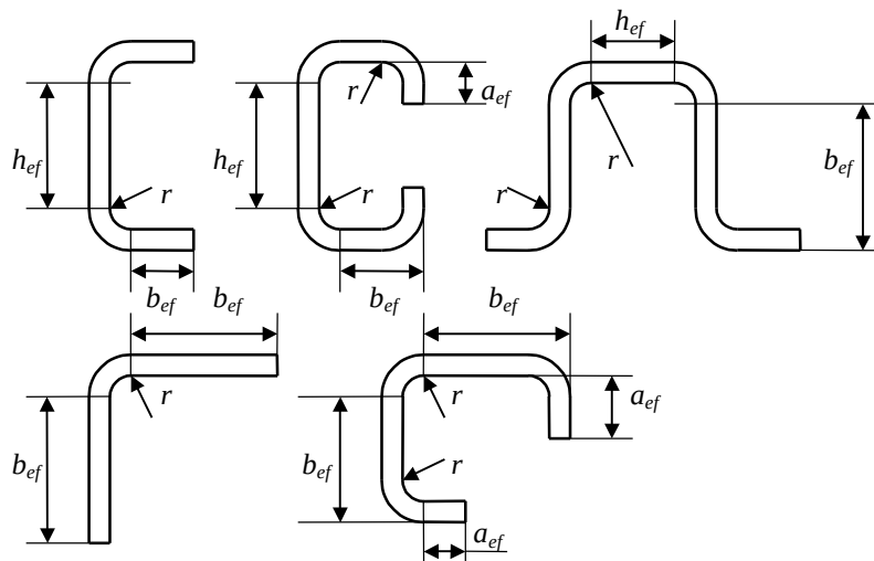
Рис. 11. Схемы поперечных сечений гнутых профилей
