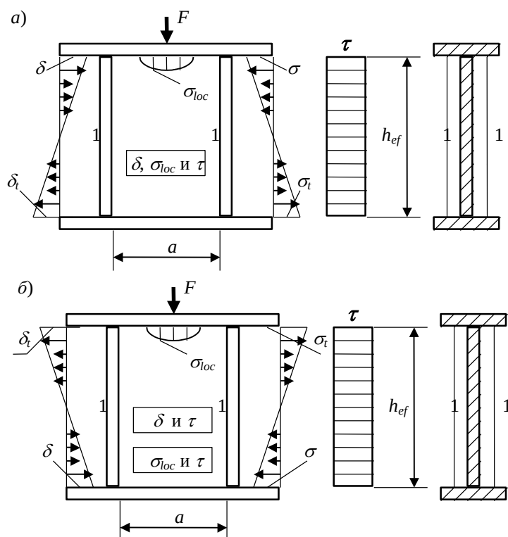
Рис. 12. Схема балки, укрепленной поперечными основными ребрами жесткости (1) а – сосредоточенная нагрузка F приложена к сжатому поясу; б – то же, к растянутому поясу
