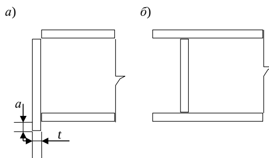
Рис. 15. Схема устройства опорного ребра жесткости a – в торце с применением строжки; б – удаленного от торца с плотной пригонкой или приваркой к нижнему поясу
