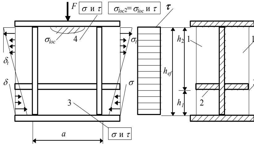
Рис. 13. Схема балки, укрепленной поперечными основными ребрами и продольным ребром жесткости
