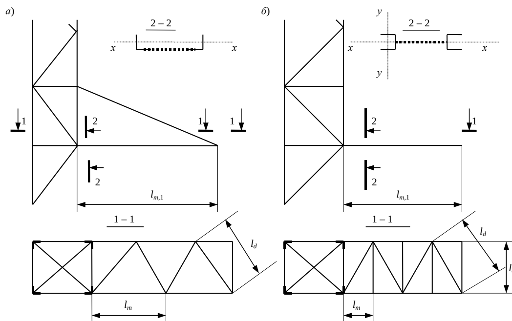
Рис. 21. Схемы траверс a – с треугольной решеткой; b – то же, со стойками
