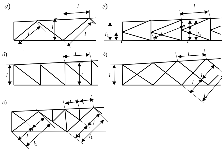
Рис. 7. Схемы решеток ферм для определения расчетных длин элементов а – треугольная со стойками; б – раскосная; в – треугольная со шпренгелем; г – полураскосная треугольная; д – перекрестная
