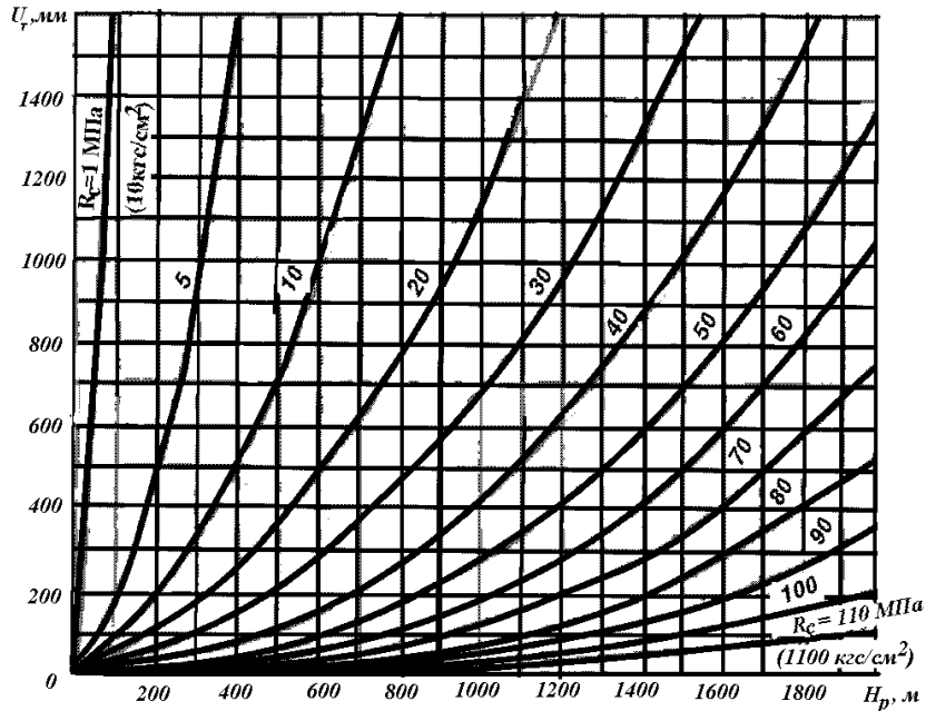
Рис. 1. Графики для определения типового смещения пород U_t
