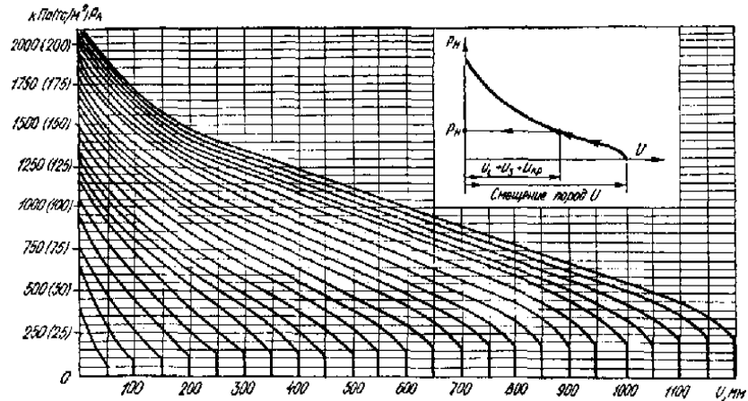
Рис. 4. Графики для определения нормативной нагрузки на крепь
