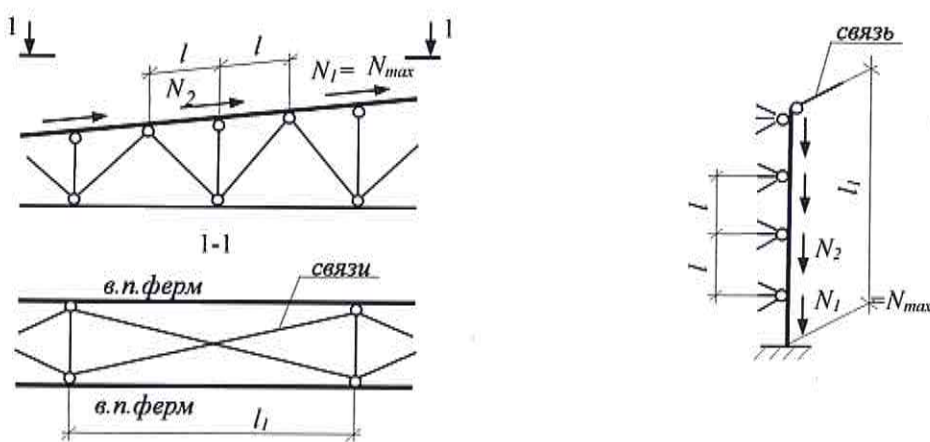
а – пояс фермы; б – ветвь колонны
