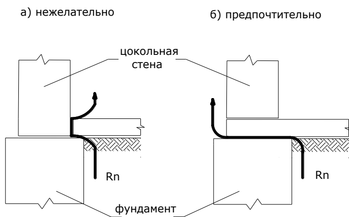
Рисунок 2 – Нерекондуемое и рекомендуемое решения узла сопряжения плиты пола с фундаментом
