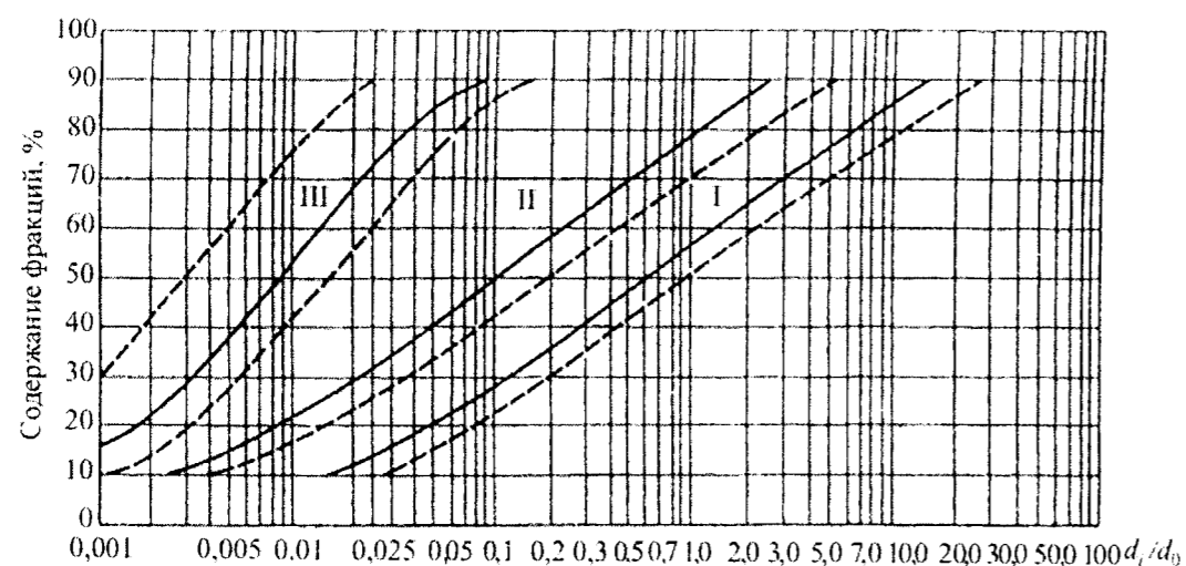
Рисунок Е.5 – График зависимости \alpha = f\left(\frac{d_i}{d_0}\right) для гравийных плотин с ядром высотой > 30 м
