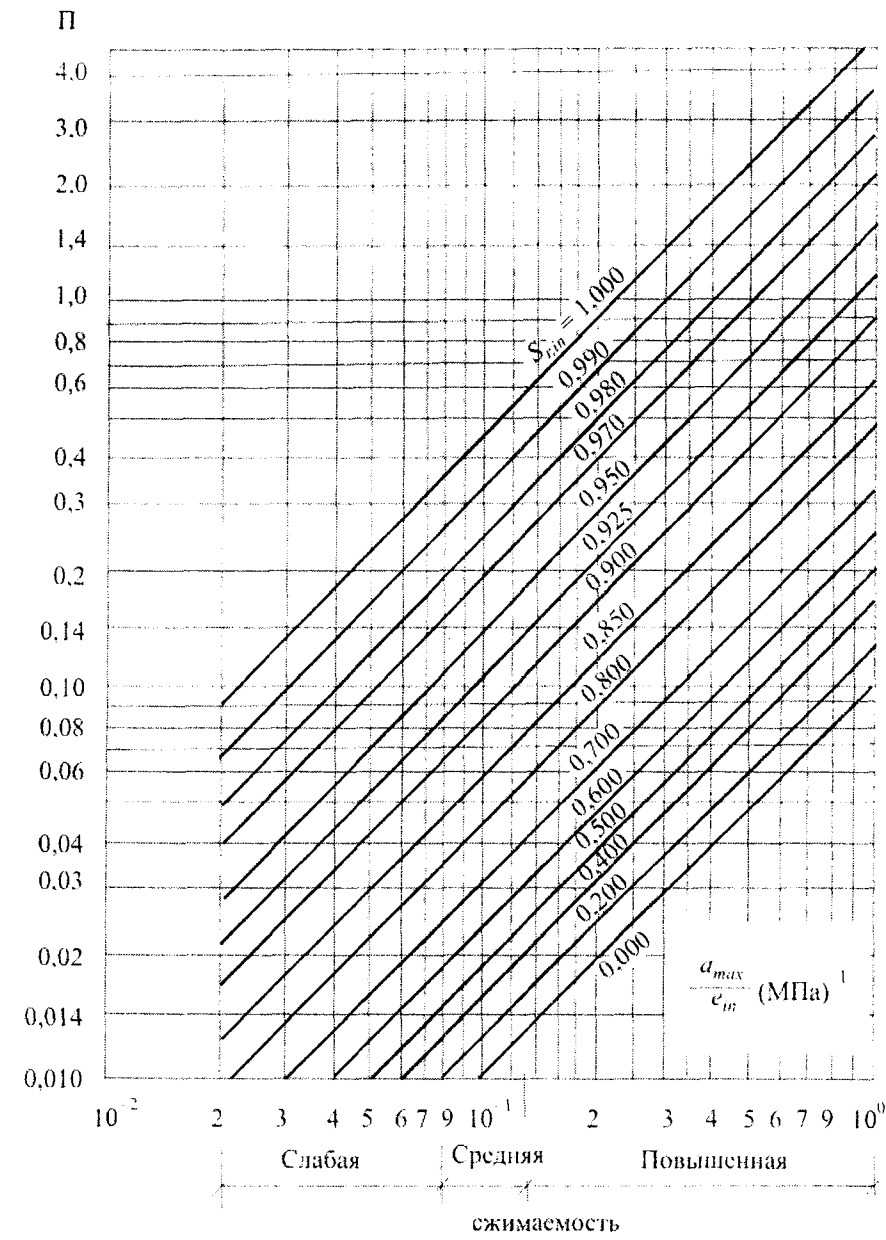
Рисунок А.2 – Номограмма для определения параметра \Pi
