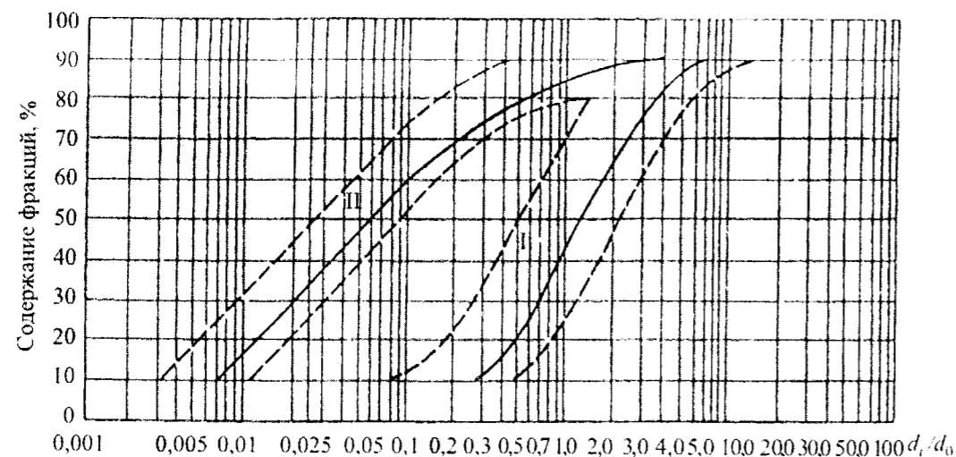
Рисунок Е.4 – График зависимости \alpha = f\left(\frac{d_i}{d_0}\right) для гравийных плотин с ядром высотой < 30 м
