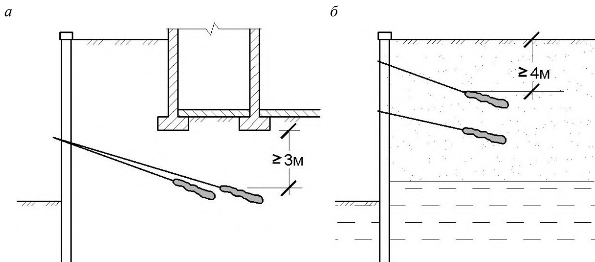
Рисунок 6.8 – Минимальное расстояние до корня анкера
