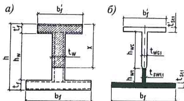
a – сечение армоцементного элемента; b – сечение, приведенное к стальному Рисунок 6.14 – Схема приведения сечения армоцементных элементов к стальному
