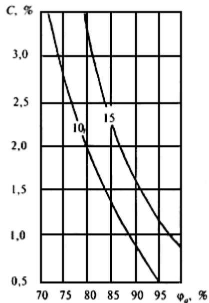
Рисунок Щ.4 - Изолинии сорбционного влагосодержания керамзитобетона \rho_0 = 1200 \text{ кг/м}^3 , содержащего NaCl - 60%, KCl - 30%, \text{MgCl}_2 - 10%, при изменении относительной влажности воздуха \varphi_a , %, и массового солесодержания C , %, в стенах флото-фабрик
