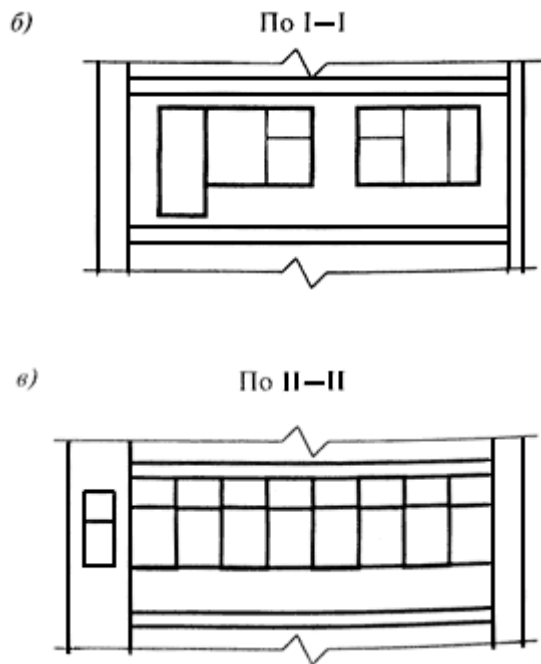
Рисунок У.1 - План (а), разрез (б) по сечению I-I плана и фасад (в) по сечению II-II остекленного балкона многоэтажного жилого здания
