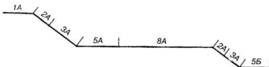
Рисунок А.5 - Схема расположения зон граничных условий на боковом откосе насыпи при наличии бермы для всех групп мостов
