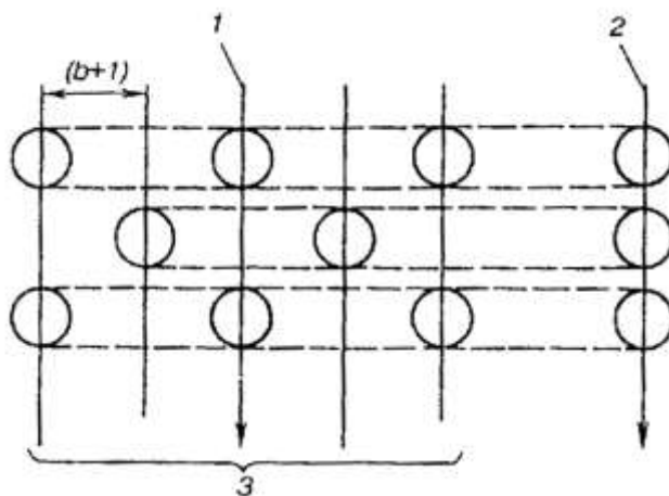
Рисунок Е.1 - Схема к определению коэффициента \kappa при шахматном расположении столбов: 1 - плоскость действия нагрузки; 2 - приведенный ряд; 3 - план расположения столбов или свай
