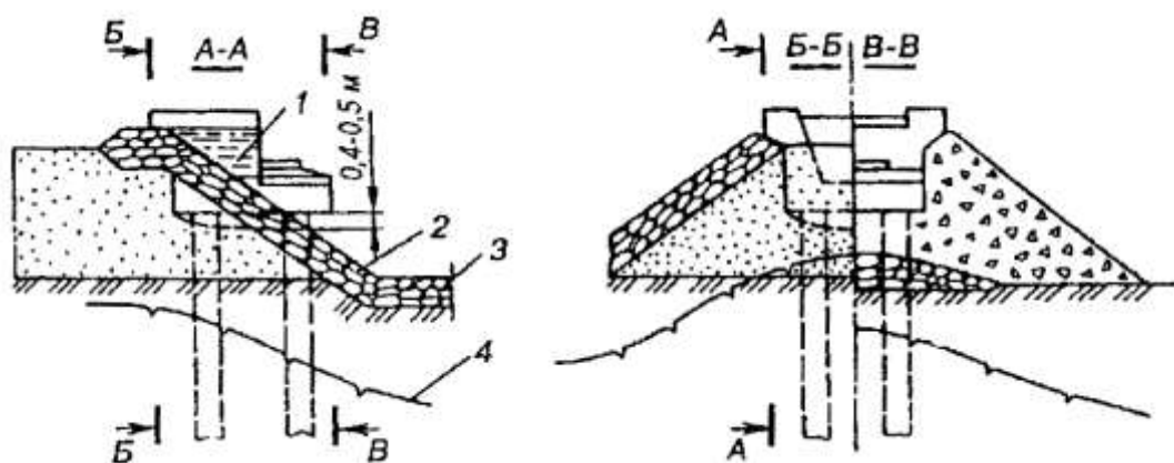
Рисунок В.4 - Схема покрытия конусов устоев наброской из камня:
