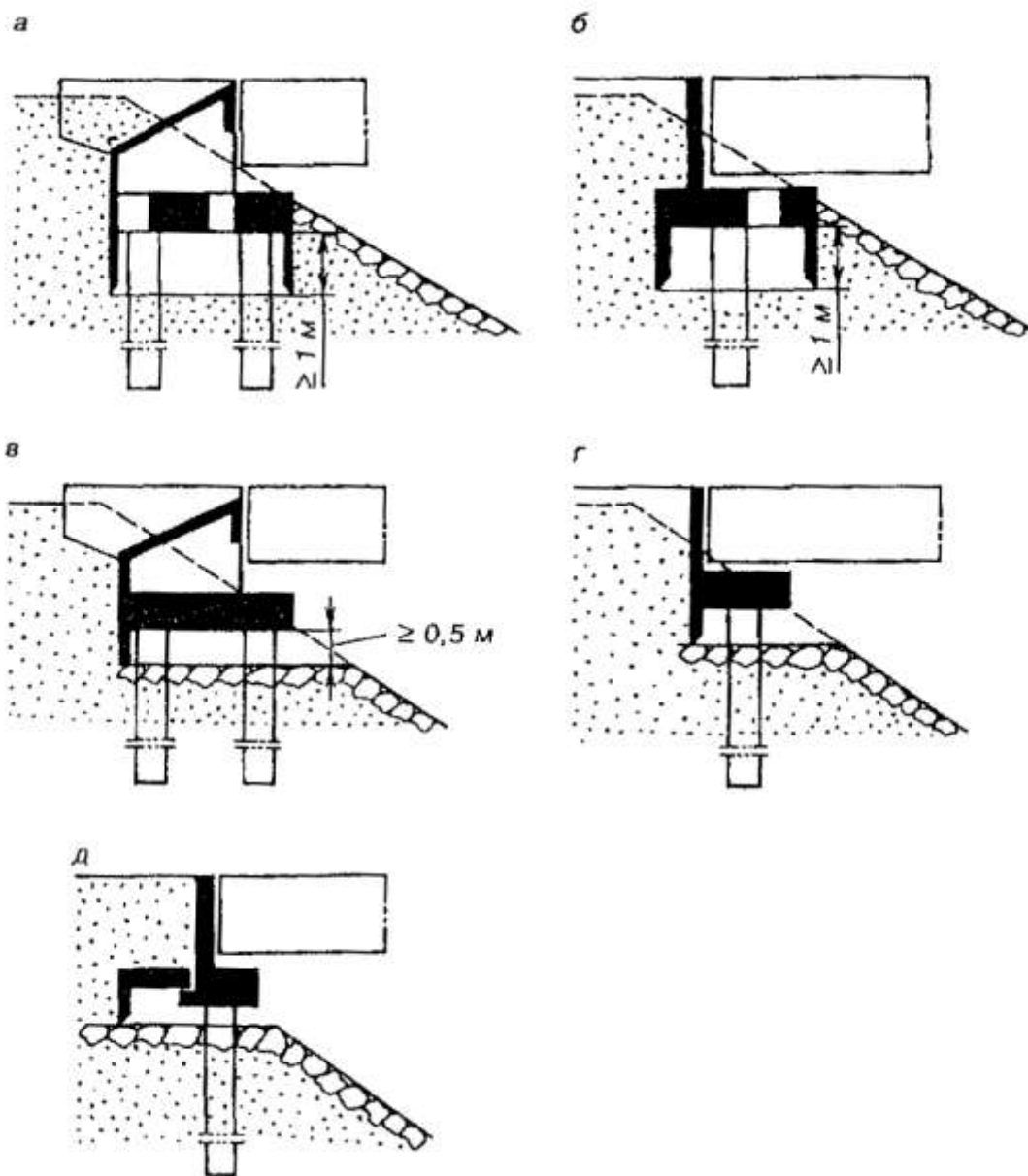
Рисунок В.2 - Схемы устройства полостей в конструкции устоев: а и б - с применением ограждающих элементов; в, г и д - увеличением зазора под насадкой
