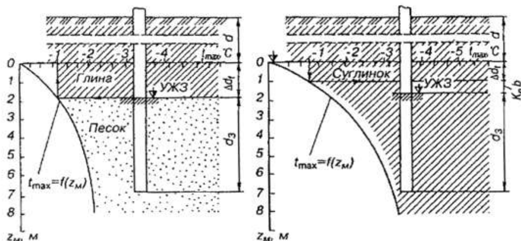
Рисунок Е.2 - График изменения расчетных температур t_{\max} по z_M (для случая расположения плиты фундамента над расчетной поверхностью грунта):
