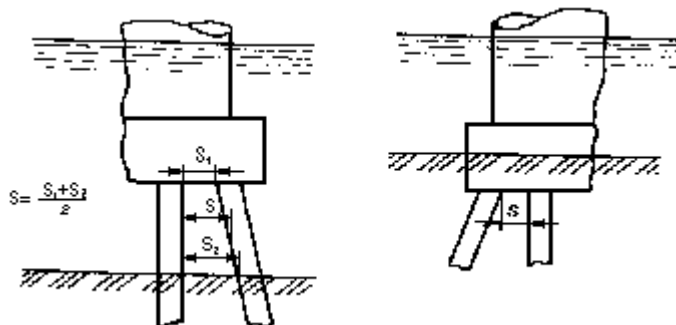
Рисунок Б.3 – Часть фасада опор с наклонными сваями фундамента
