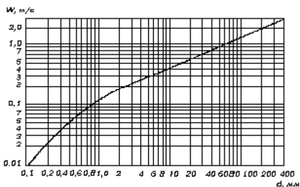
Рисунок А.3 – График для определения гидравлической крупности несвязных грунтов
