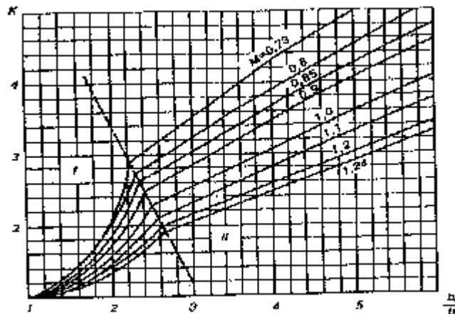
Рисунок 5.7 – График для определения коэффициента косины K
