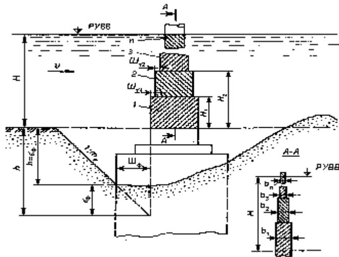
Рисунок 5.3 – Разделение опоры на элементы (1, 2, 3, ... n ) с постоянной шириной
