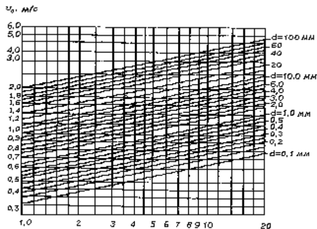
Рисунок А.1. – График для определения размывающей скорости несвязных грунтов
