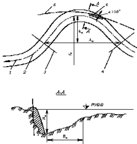
Рисунок Т.1 – К определению радиуса кривизны потока r_n :
