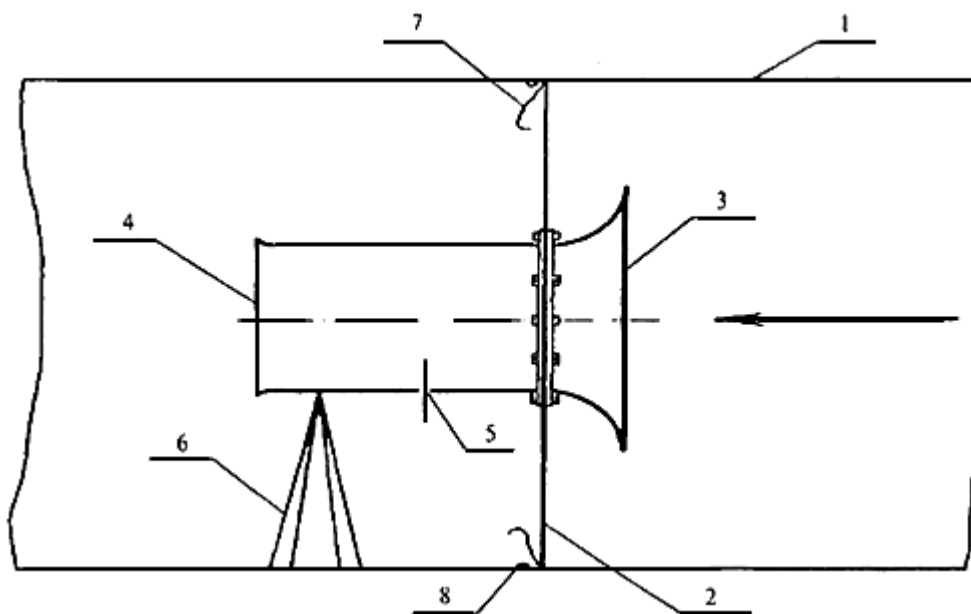
1 - вентиляционный тоннель; 2 - перемычка; 3 - входной раструб; 4 - цилиндрическая часть; 5 - отверстие для установки измерительного прибора; 6 - штатив; 7- крепежные устройства (тесемки, ремень); 8 - решетка
