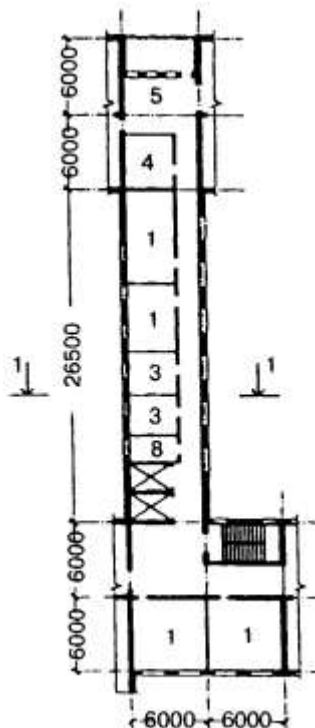
Фрагмент плана 3-го этажа
