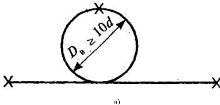
Рисунок 5 — Устройство компенсаторов П-образного (а), Г-образного (б), петлеобразного (в)
