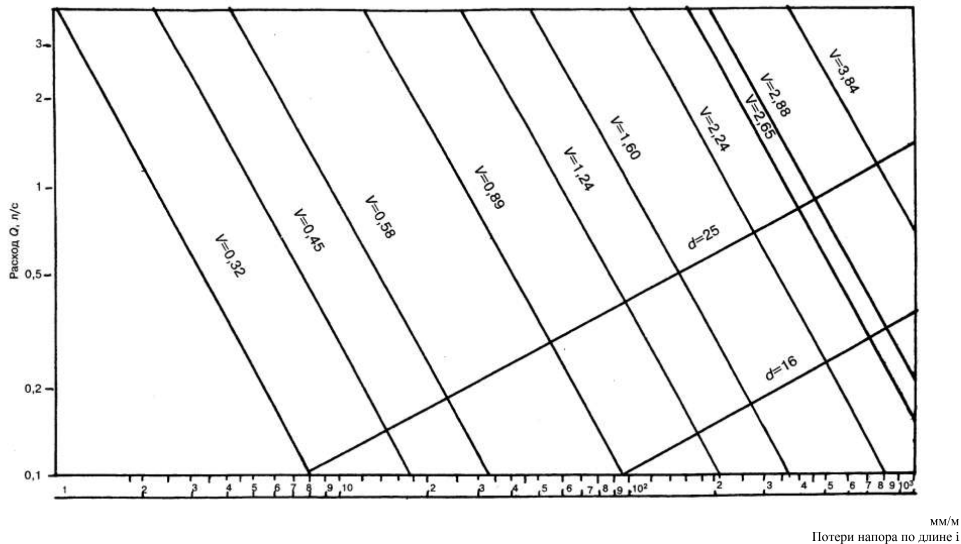
Рисунок А.1 - Номограмма для приближенного гидравлического расчета водопровода горячей воды из металлополимерных труб по ТУ 2248-004-07629379-97
