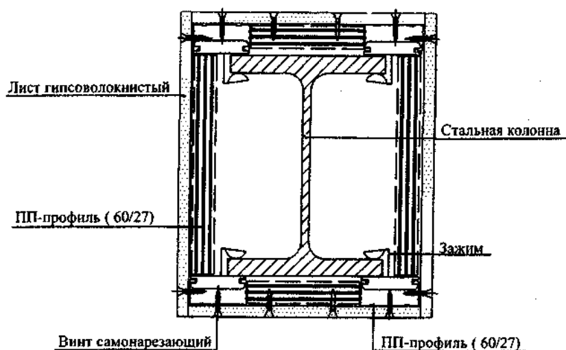
Рисунок 16 — Общий вид (а), конструктивное решение огнезащиты деревянной балки (б, з) и колонны (в)
