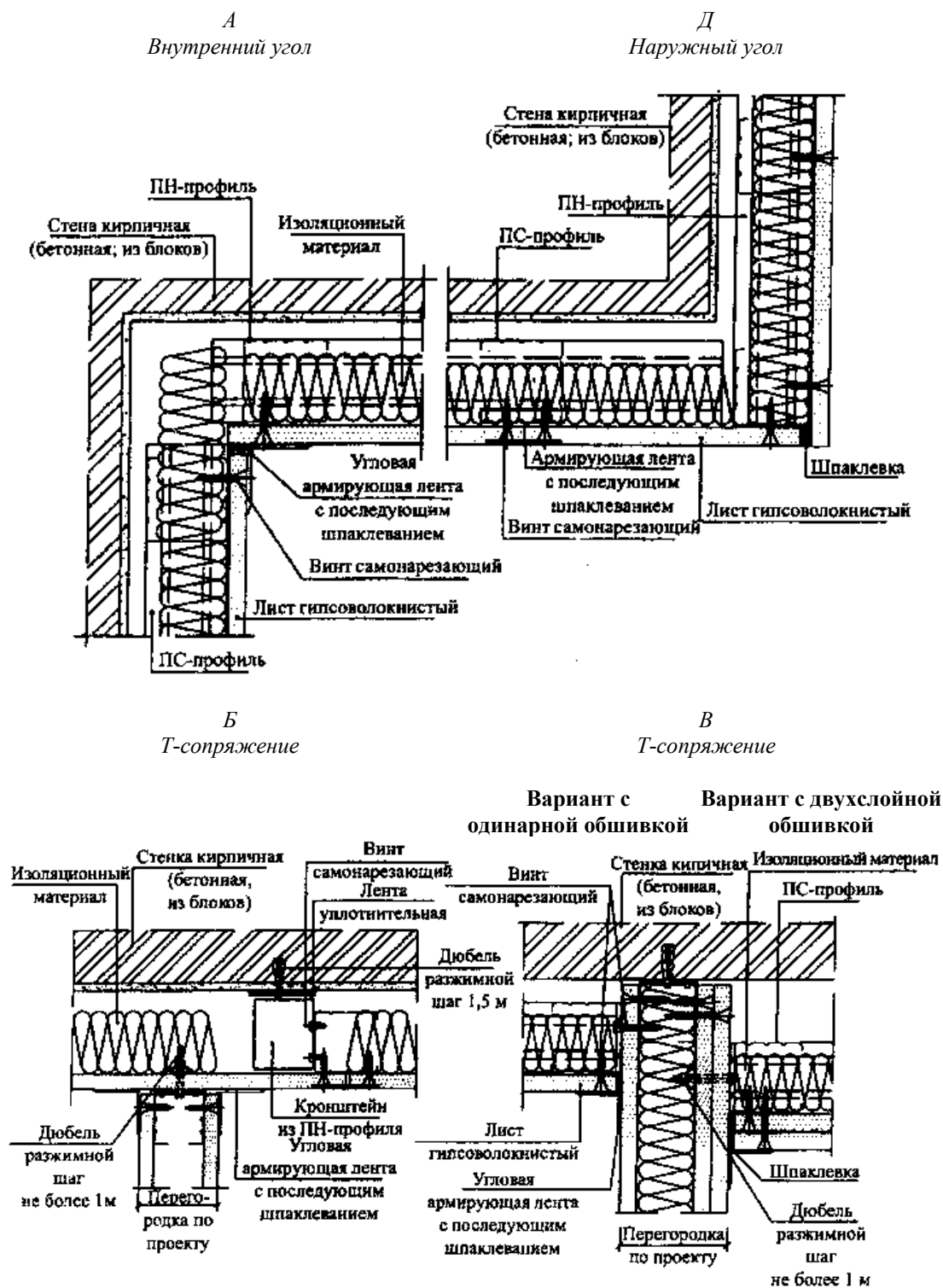
Рисунок 8 — Горизонтальный и вертикальный разрезы, узлы примыканий, внутренние и внешние углы облицовки с одинарной обшивкой гипсоволокнистыми листами по металлическому каркасу
