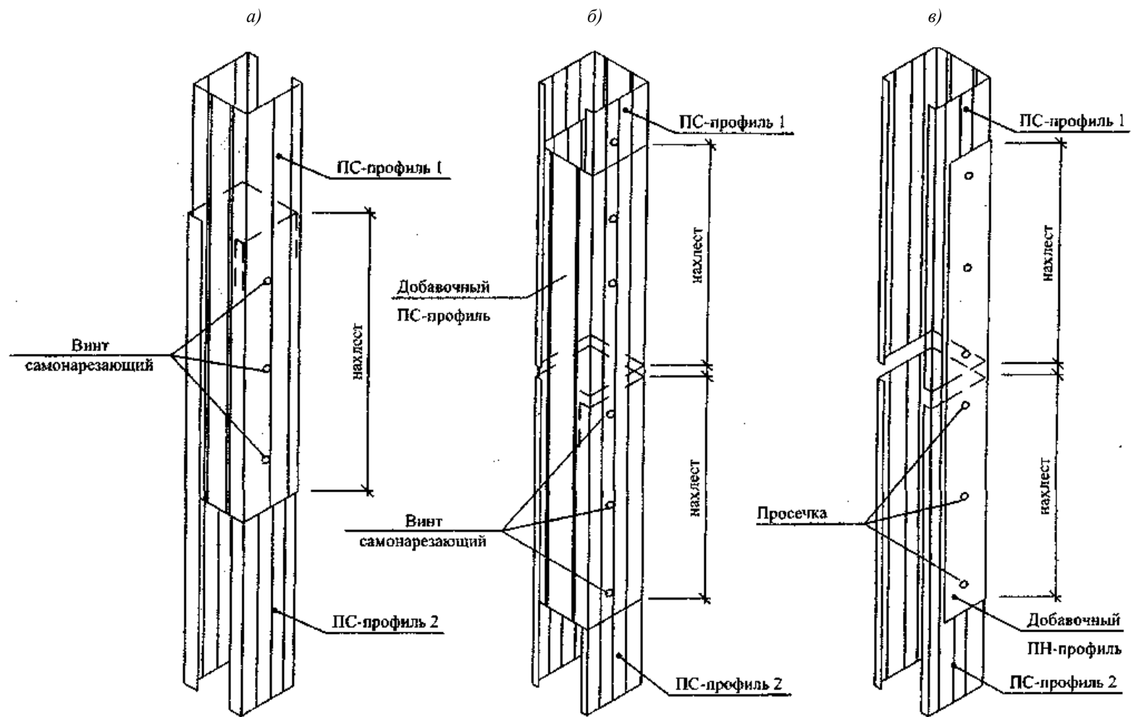
Рисунок 1 — Соединение металлических профилей методом насадки (а) и встык с дополнительным профилем (б и в)
