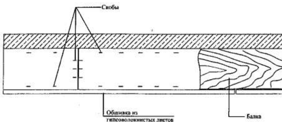
Рисунок 16 — Общий вид (а), конструктивное решение огнезащиты деревянной балки (б, з) и колонны (в)
