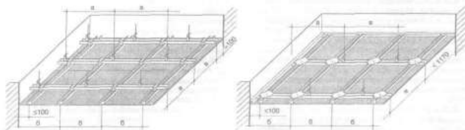
1 — конструкция двухуровневого потолка; 2 — конструкция одноуровневого потолка; a — расстояние между подвесами, b — расстояние между несущими профилями, в — расстояние между основными профилями Рисунок 13 — Конструкции подвесных потолков
