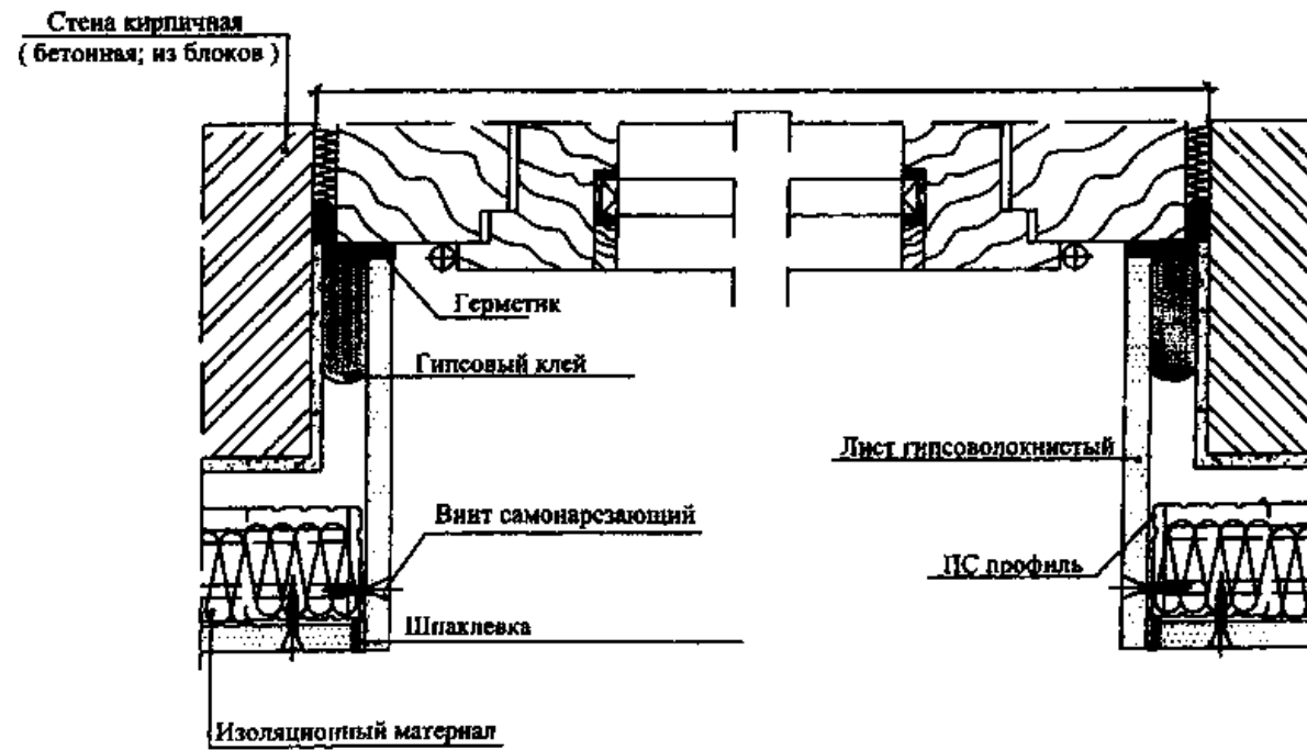
Рисунок 9 — Температурные швы, оконный или дверной проем при облицовке стен
