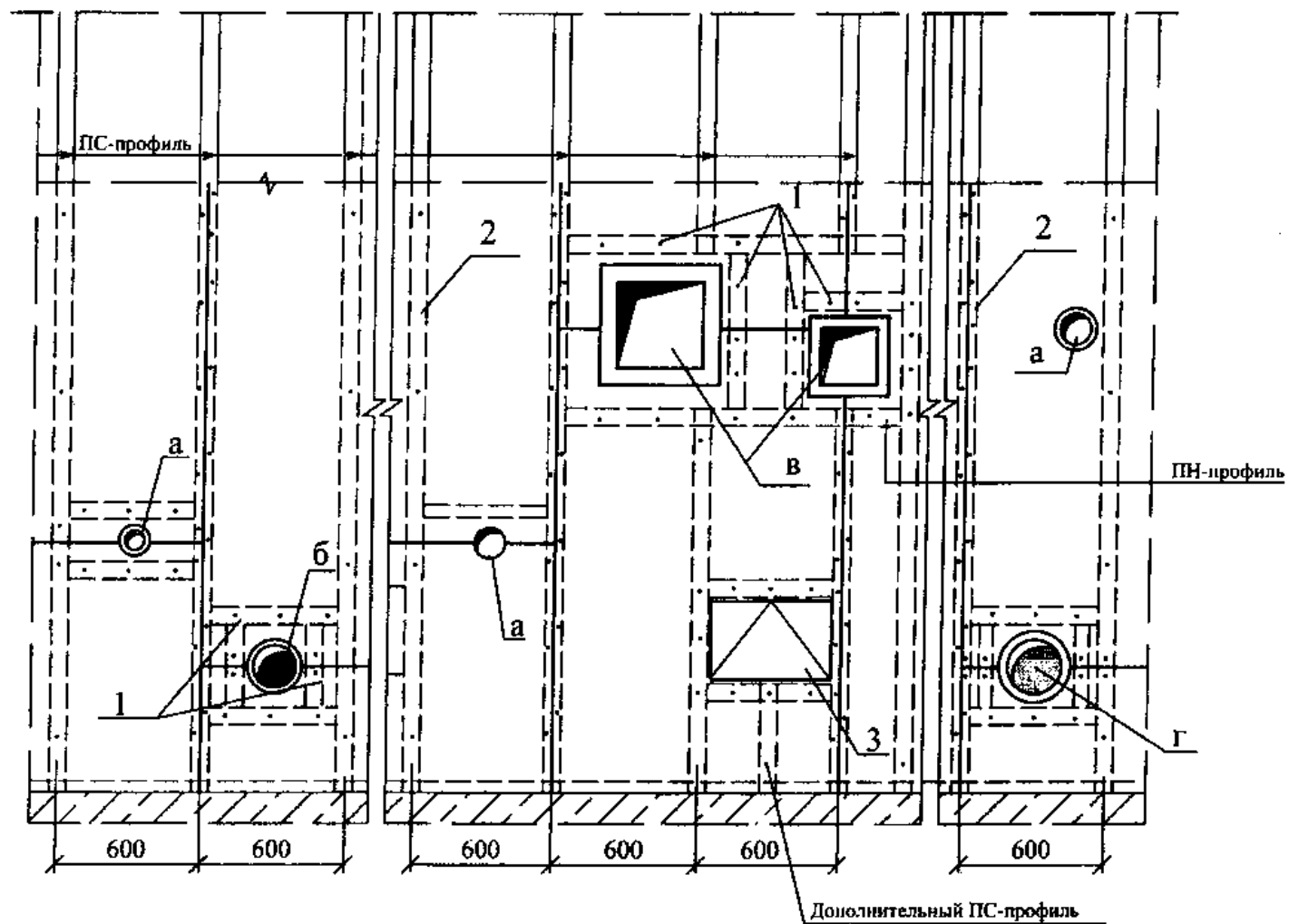
1 — обрамляющие элементы; 2 — дополнительная стойка; 3 — ревизионный люк Рисунок 5 — Схема размещения трубопроводов диаметром не более 60 мм (а), технологических трубопроводов — не менее 60 мм (б), воздухопроводов (в) и трубопроводов водоснабжения и отопления (г)
