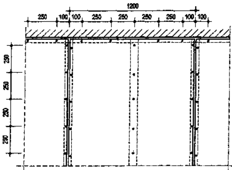
Рисунок 18 — Крепление гипсоволокнистых листов к каркасу
