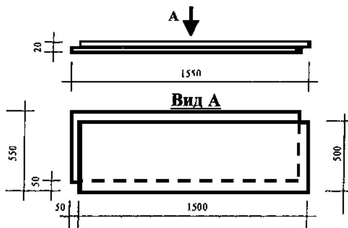
Рисунок 14 — Элемент сборного основания пола
