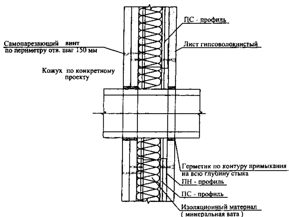
Рисунок 7 - Схема устройства гильзы (а) и кожуха (б) при сопряжении перегородки из гипсоволокнистых листов с трубопроводами
