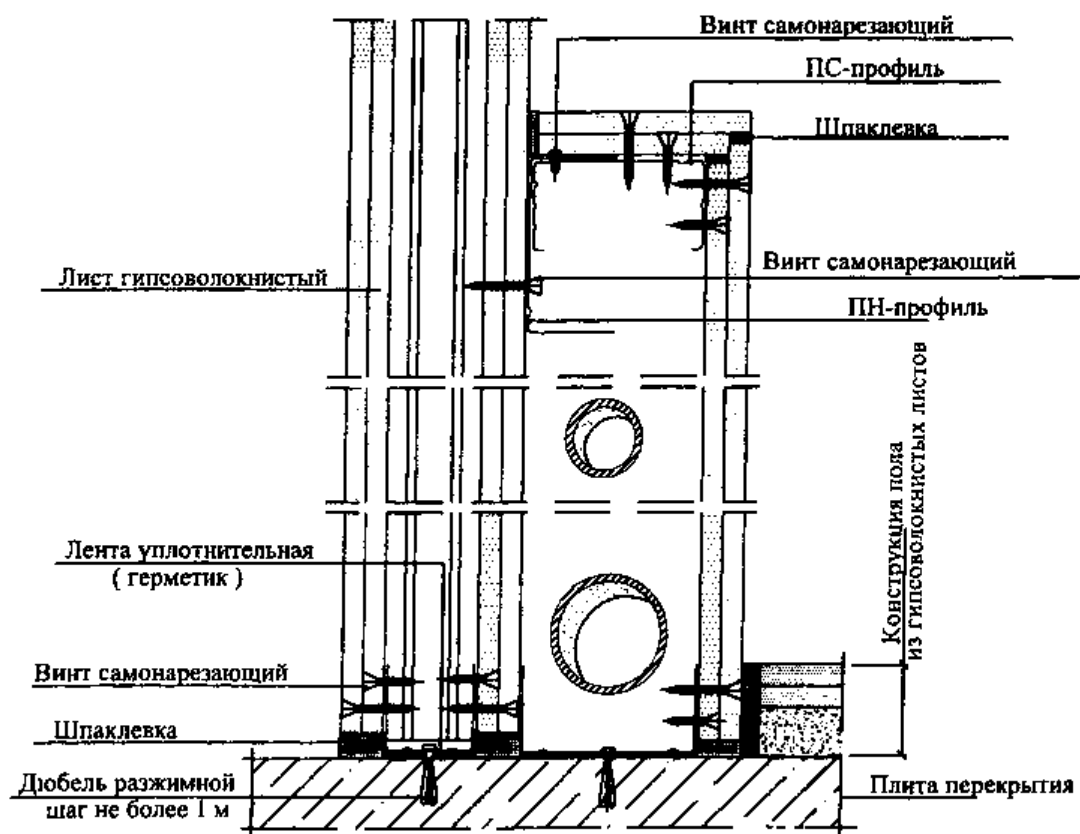
Рисунок 10 — Конструктивное решение оформления трубопроводов, размещенных вдоль капитальной стены (а), перегородки (б)
